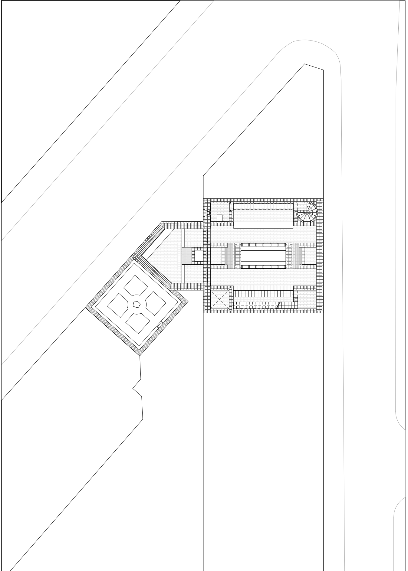
Grundriss 1 M 1:200
