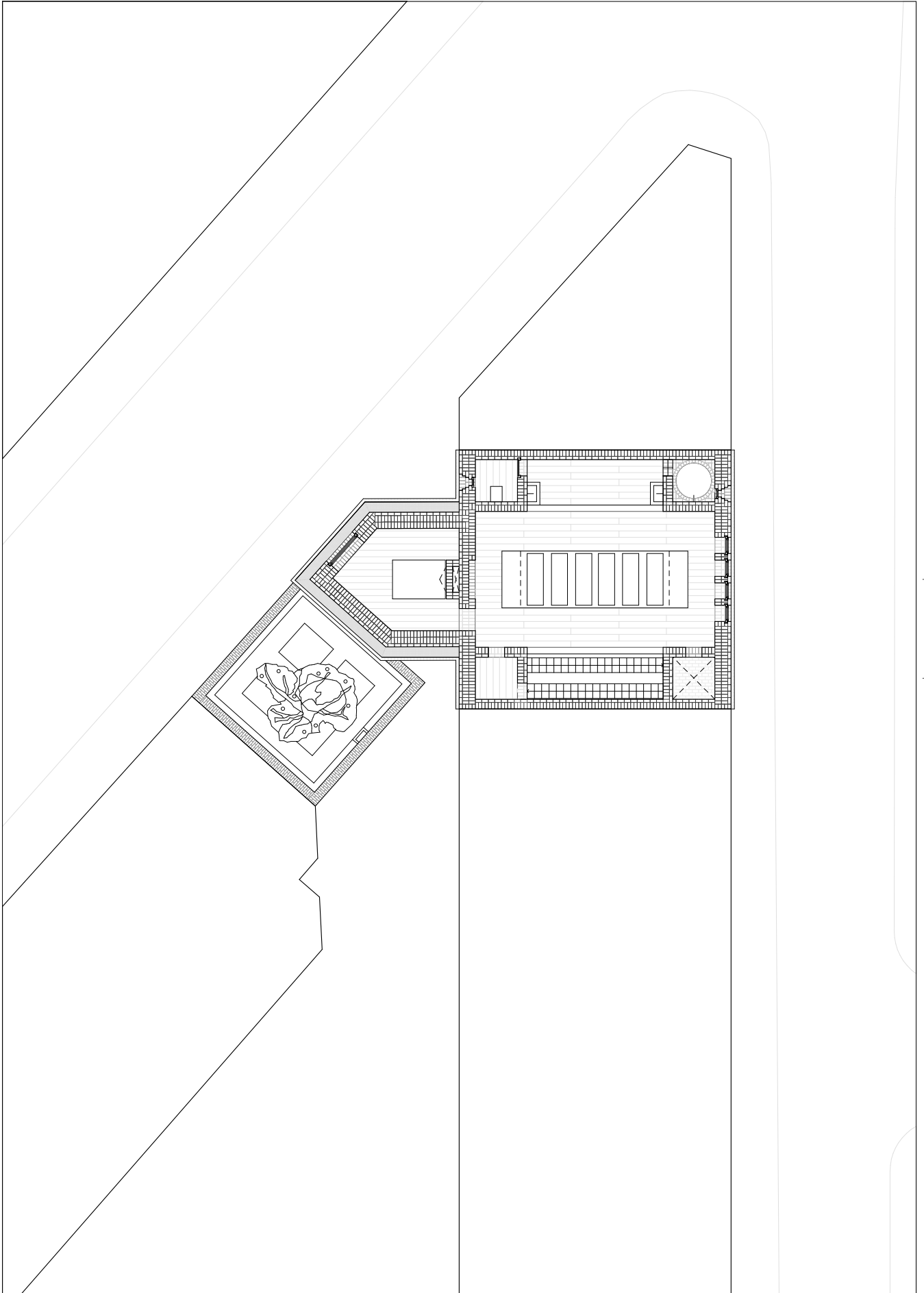
Grundriss 2 M 1:200
