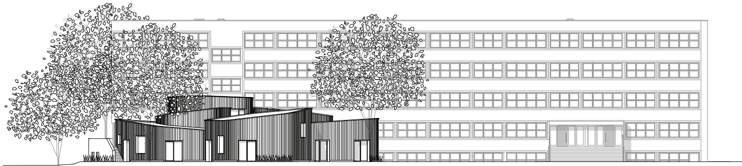
Ansicht Südost
