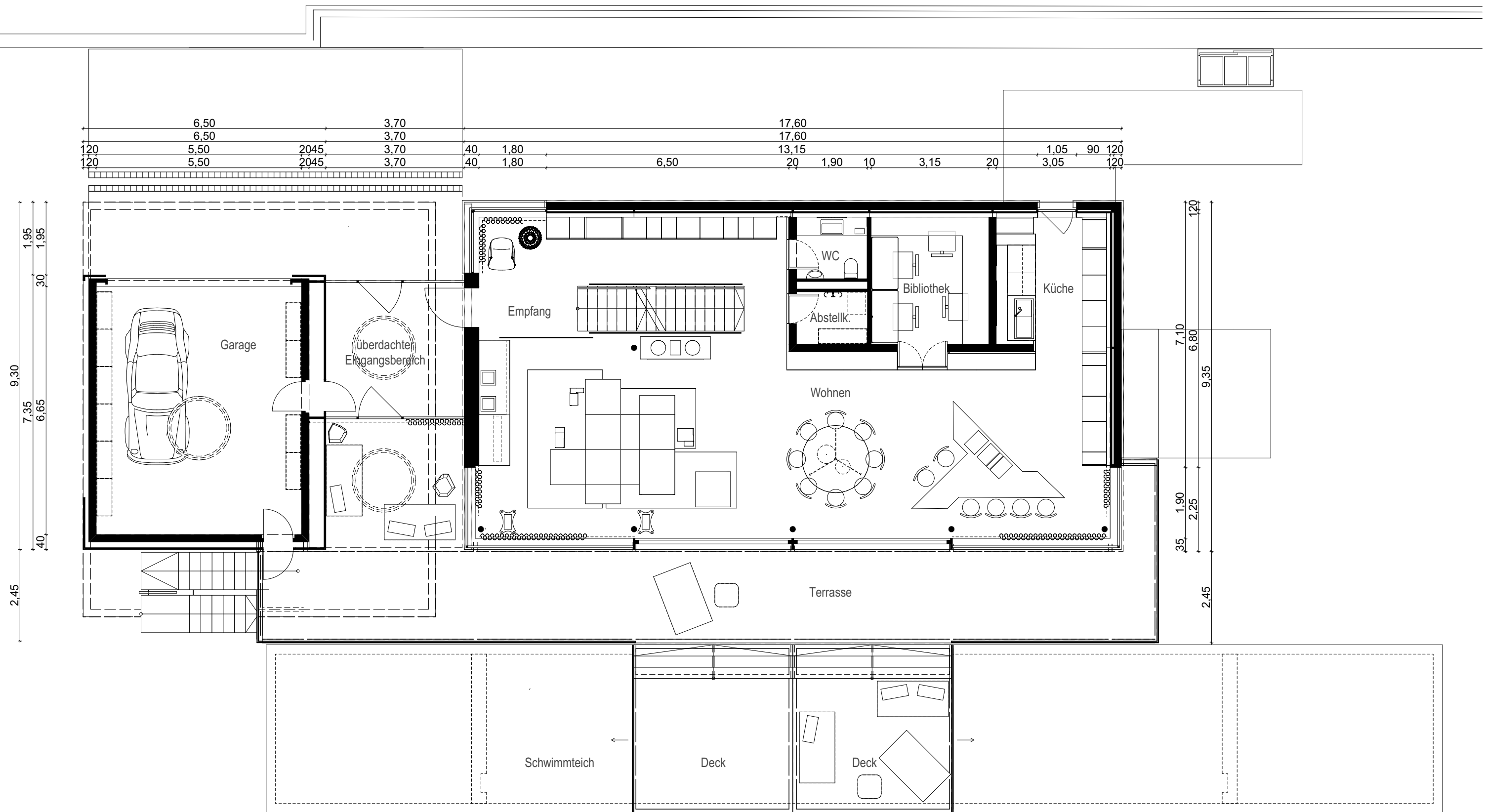
Grundriss Erdgeschoss M1:100
