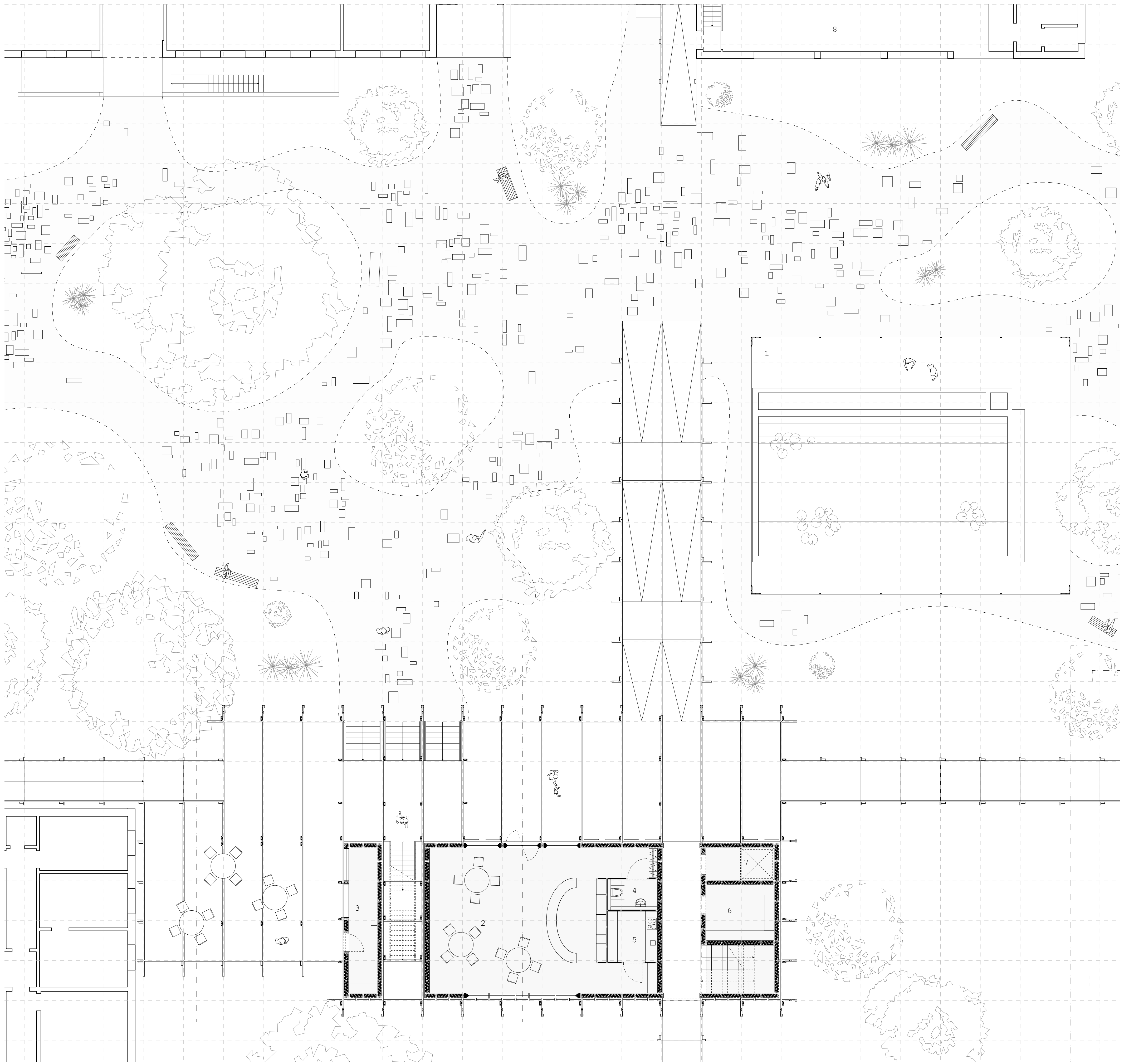
Grundriss EG Meditation 1:100
