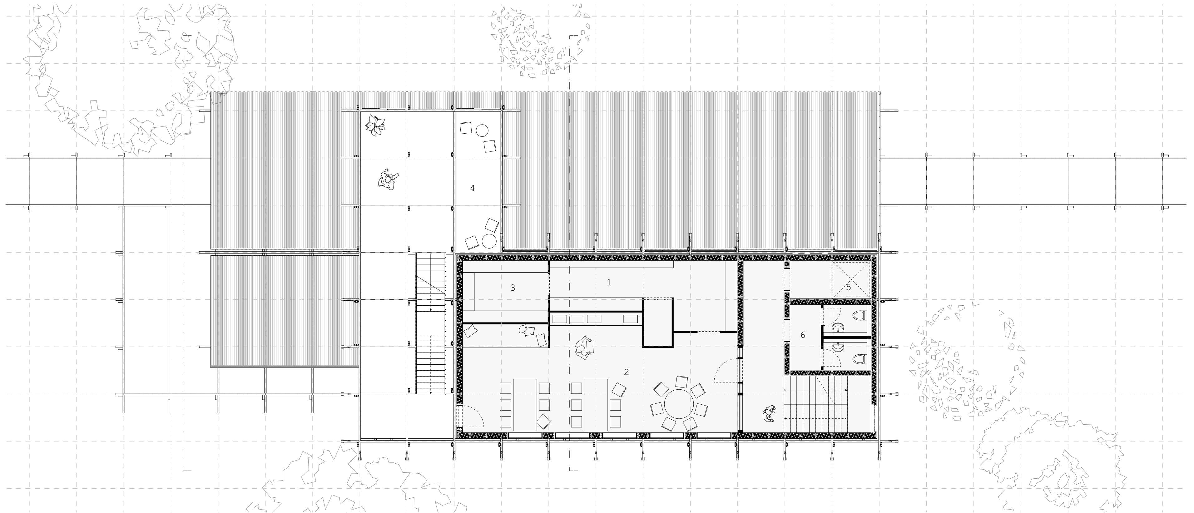
Grundriss 1.OG Meditation 1:100
