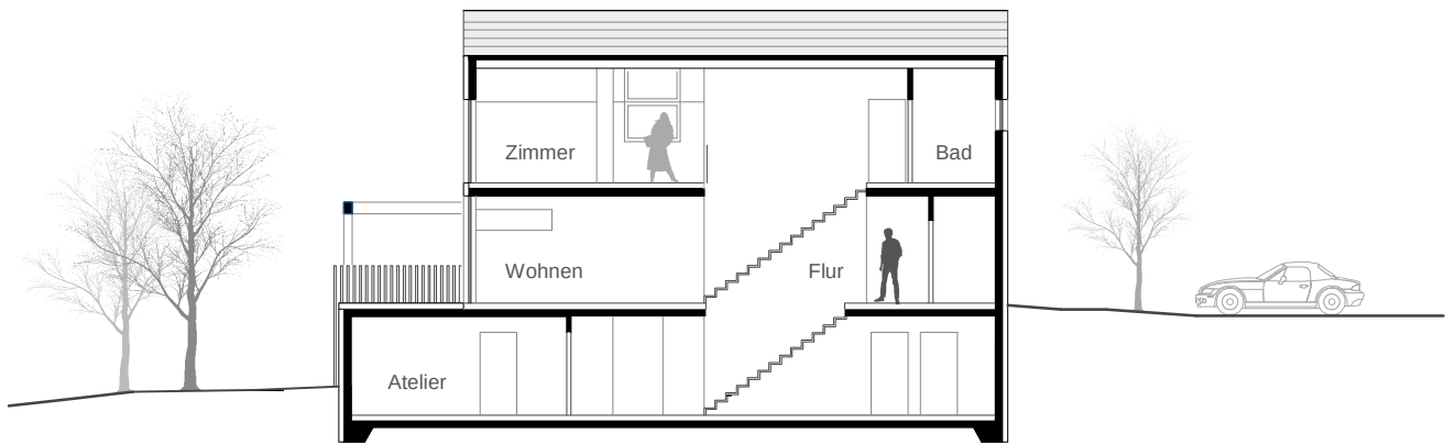
LÄNGSSCHNITT
