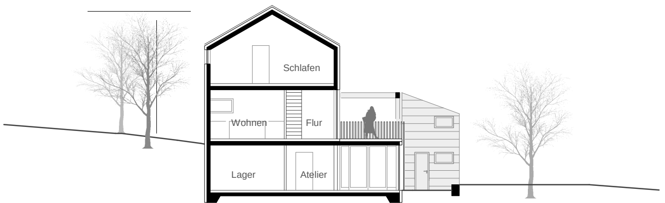
QUERSCHNITT
