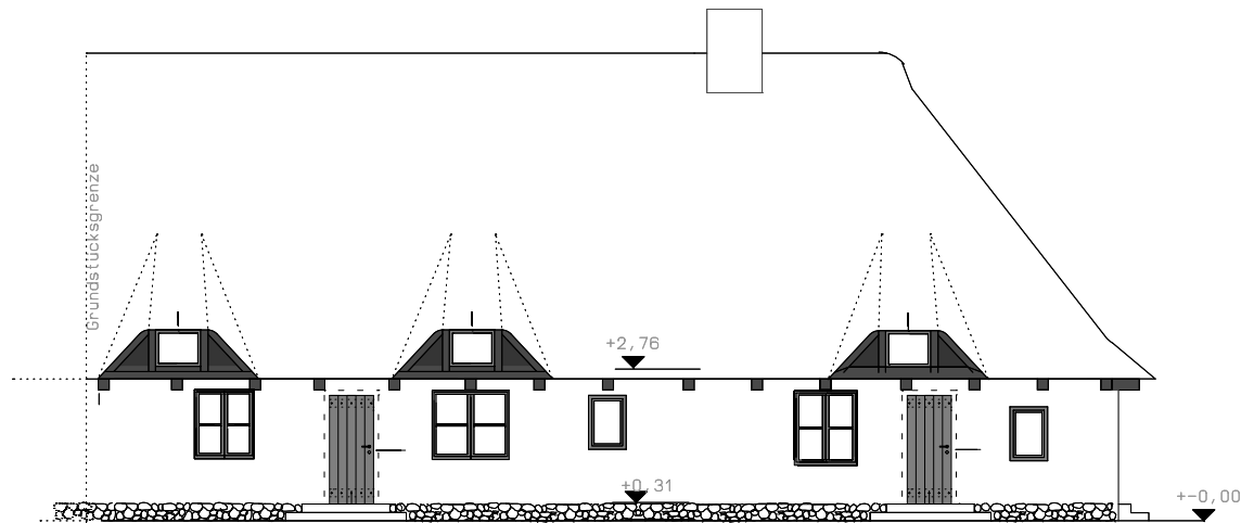
Ansicht Strasse
