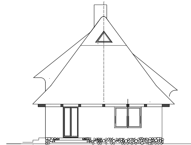
Ansicht Stirnseite
