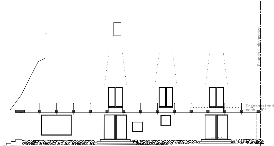
Ansicht Garten
