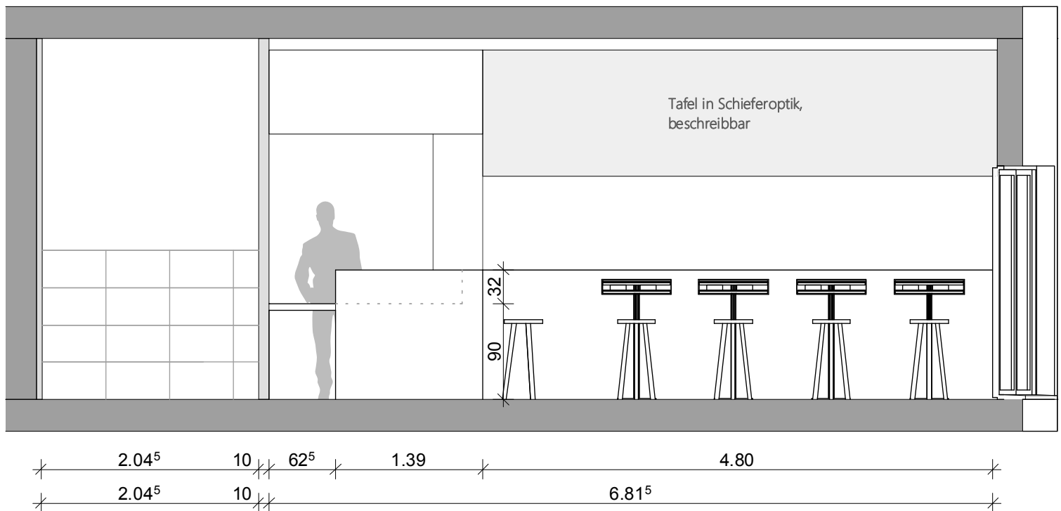
Schnitt D
