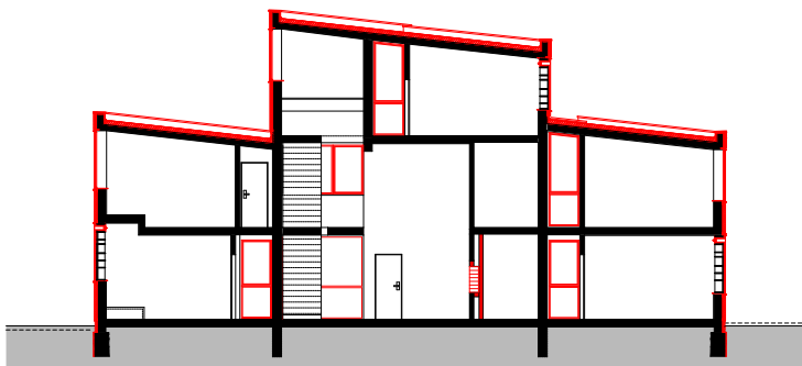
HAUS 23 – SCHNITT C-C
