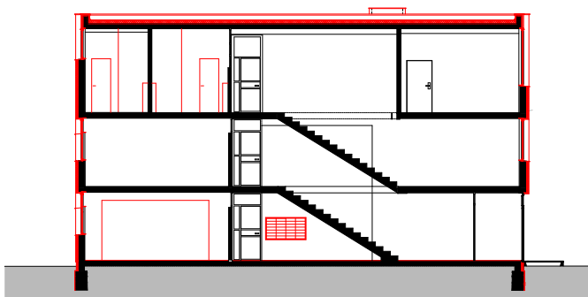
HAUS 22 – SCHNITT B-B
