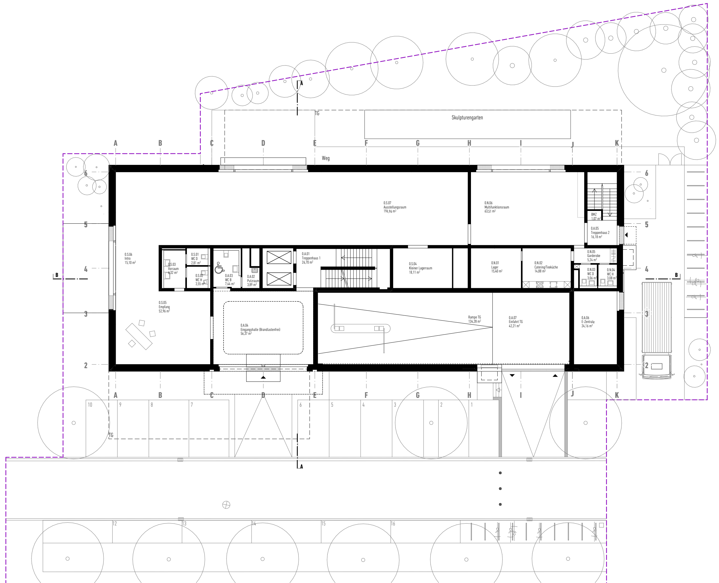
Grundriss EG
