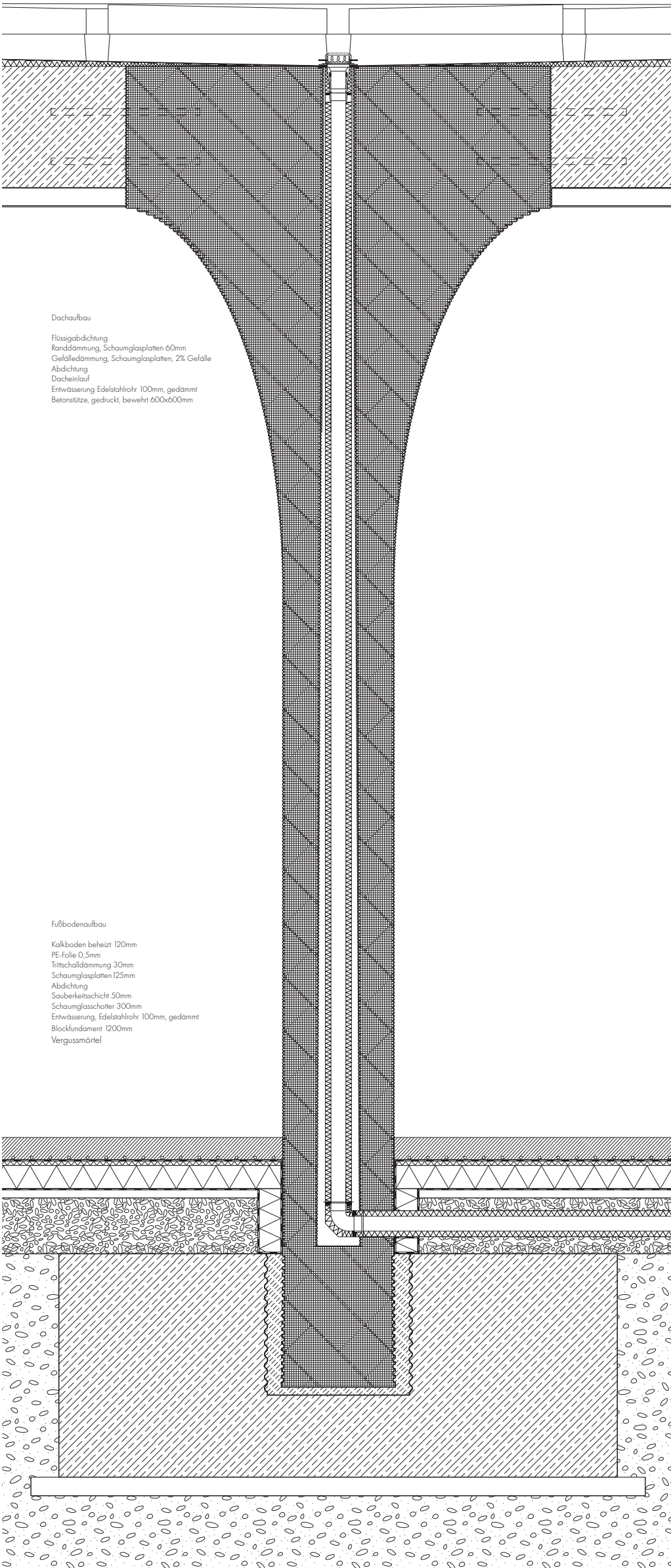
Detail C - C Stütze M 1:20
