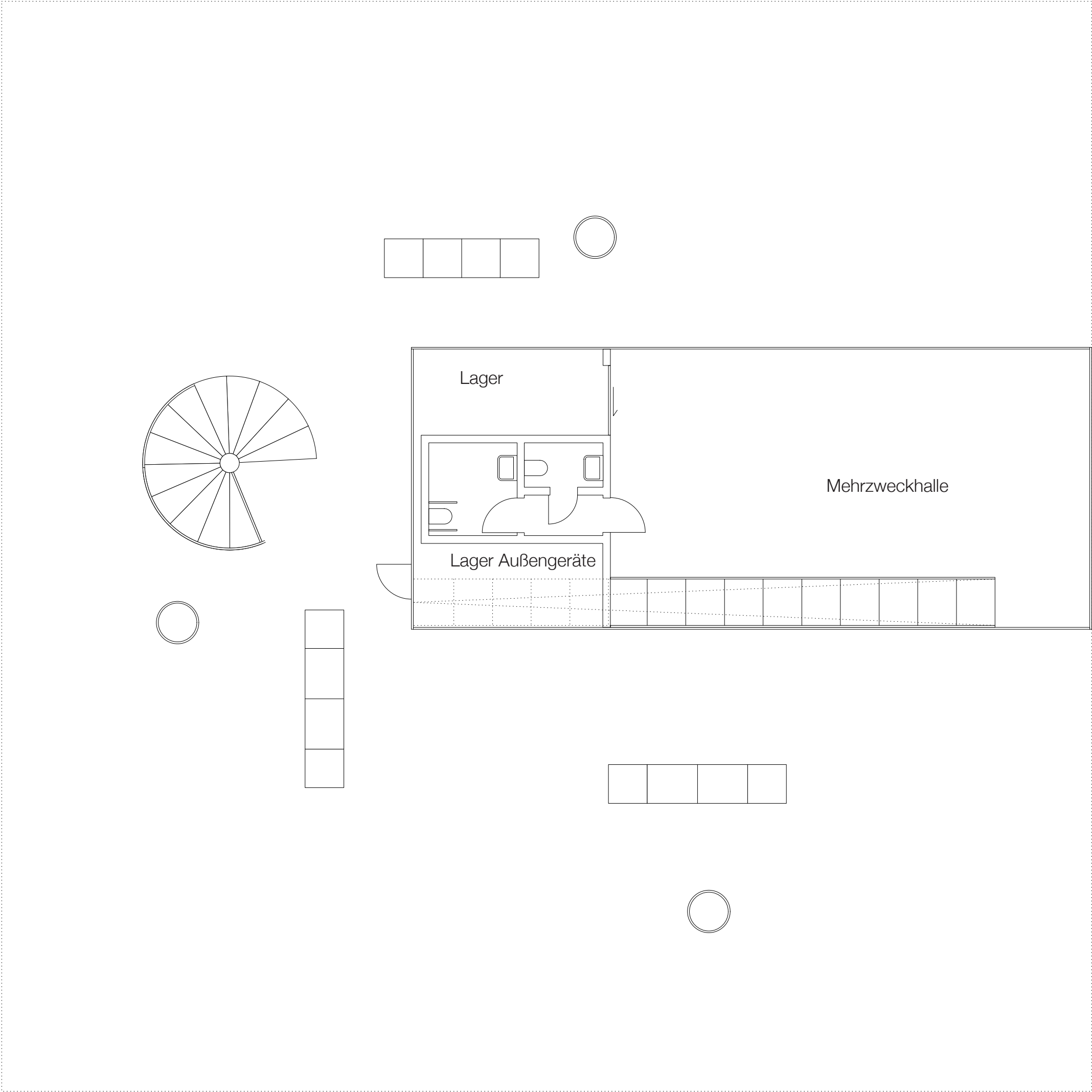
Grundriss EG 1.100
