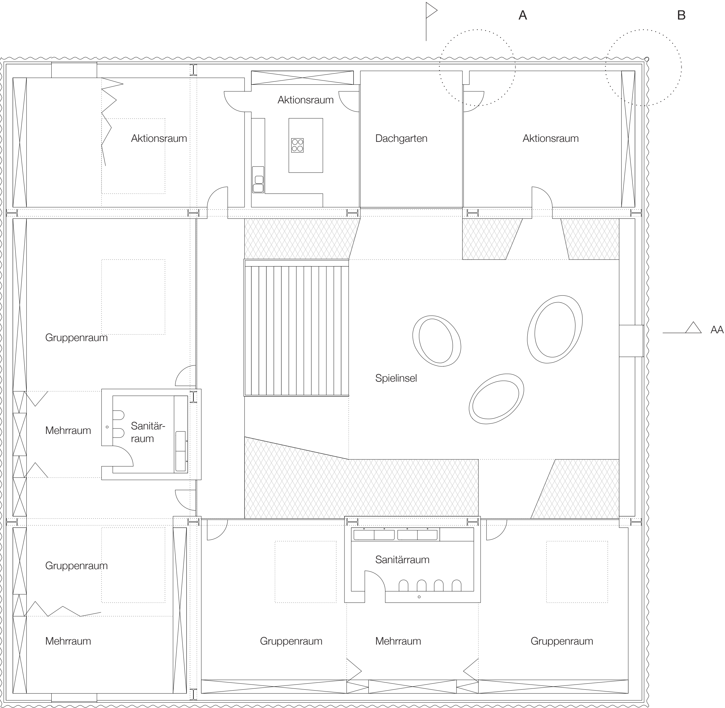
Grundriss 2. OG 1.100
