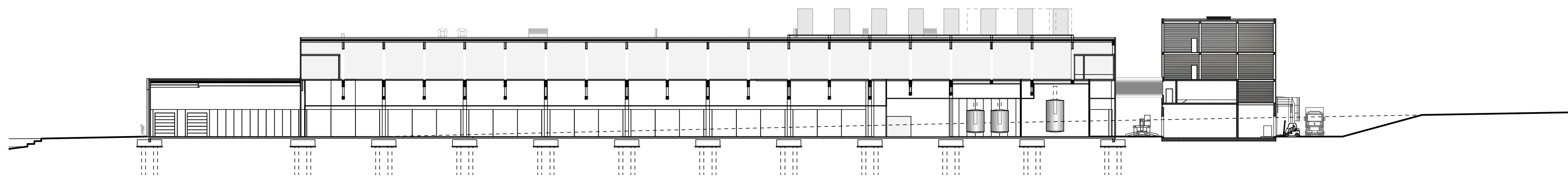
Längsschnitt Versand
