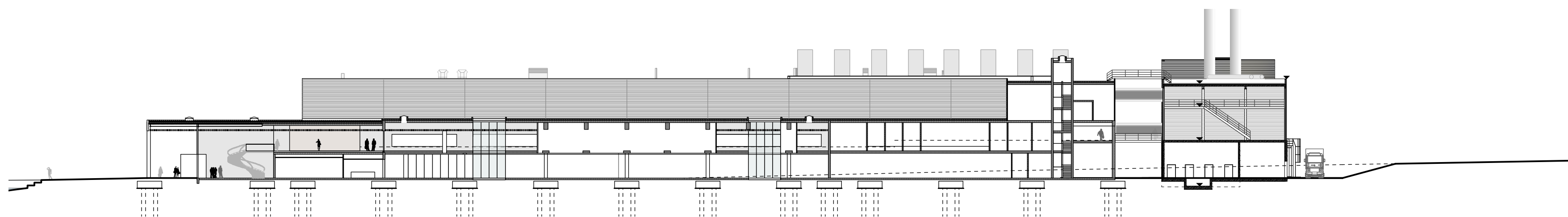
Längsschnitt Besuchergang
