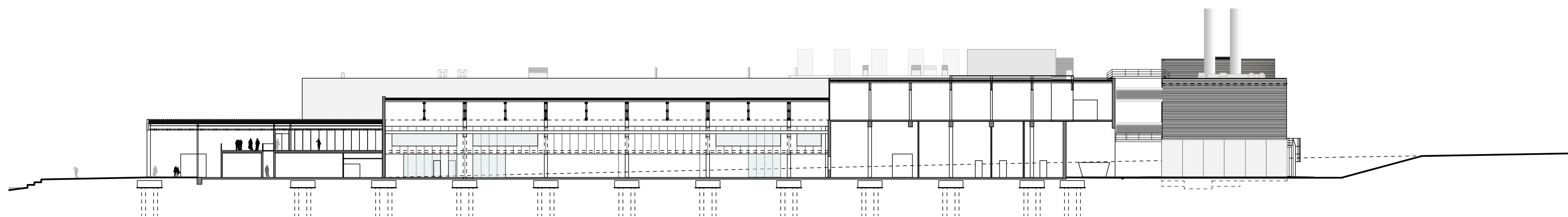
Längsschnitt Foyer
