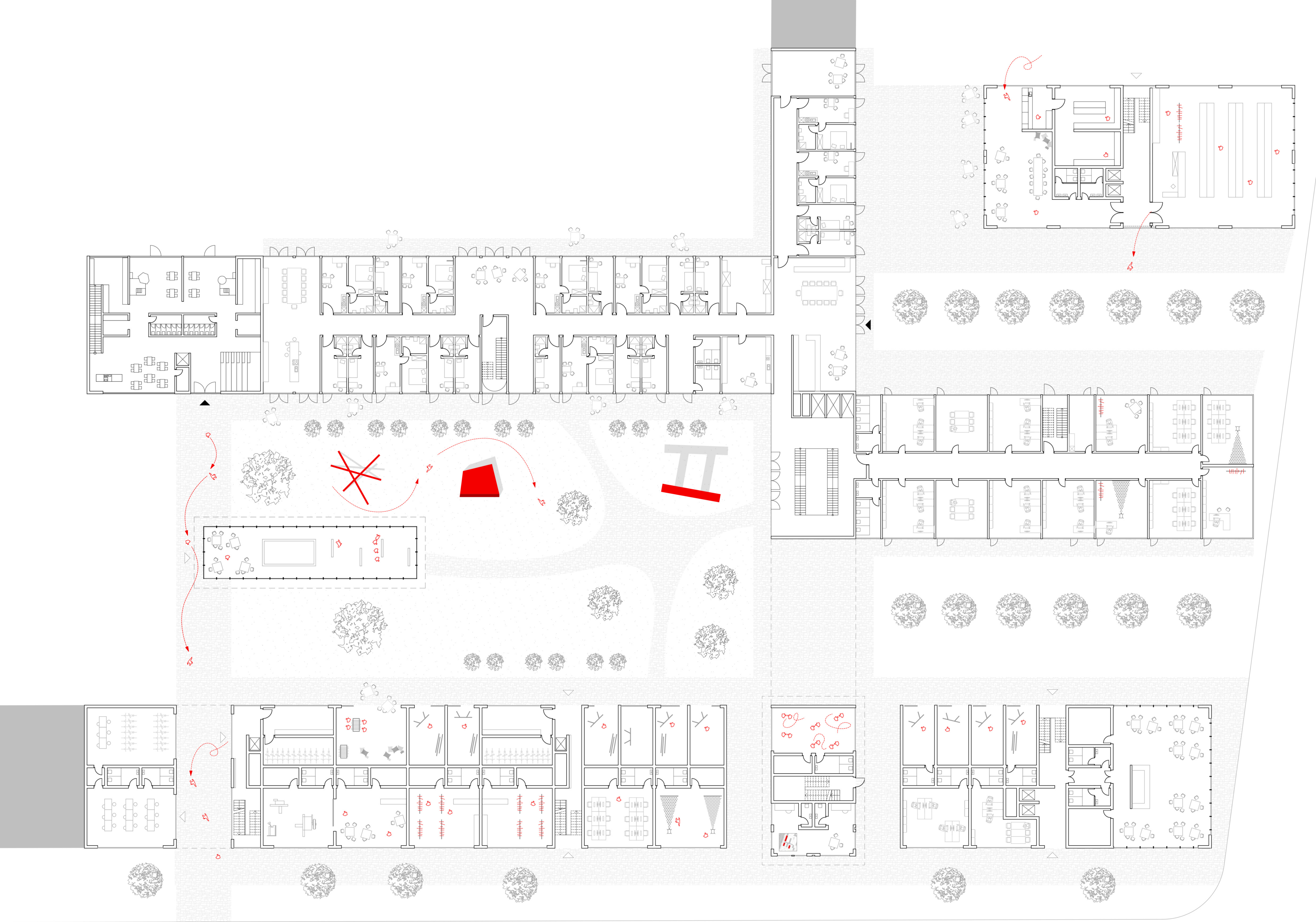
Grundriss EG M 1 : 200
