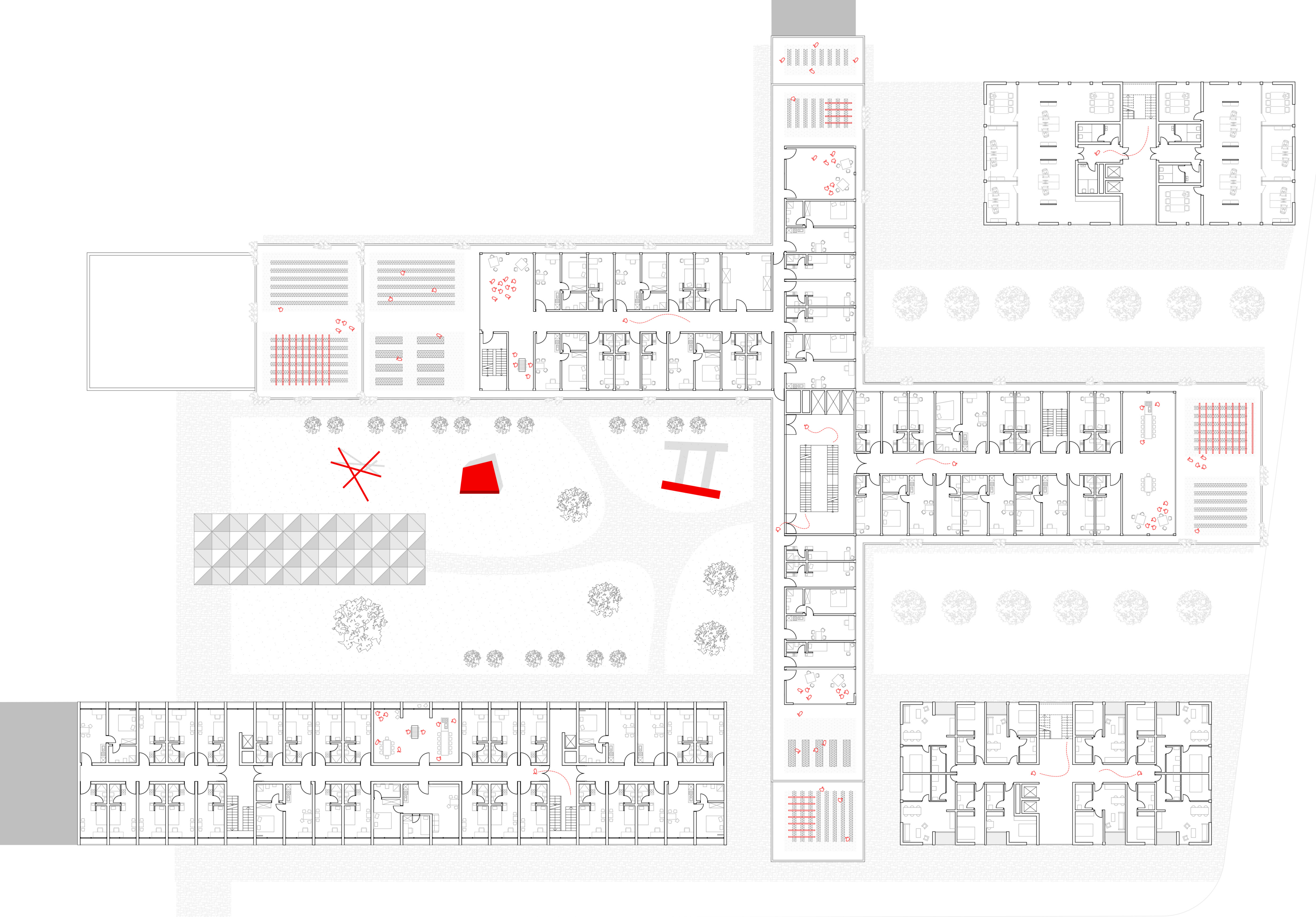
Grundriss OG M 1 : 200
