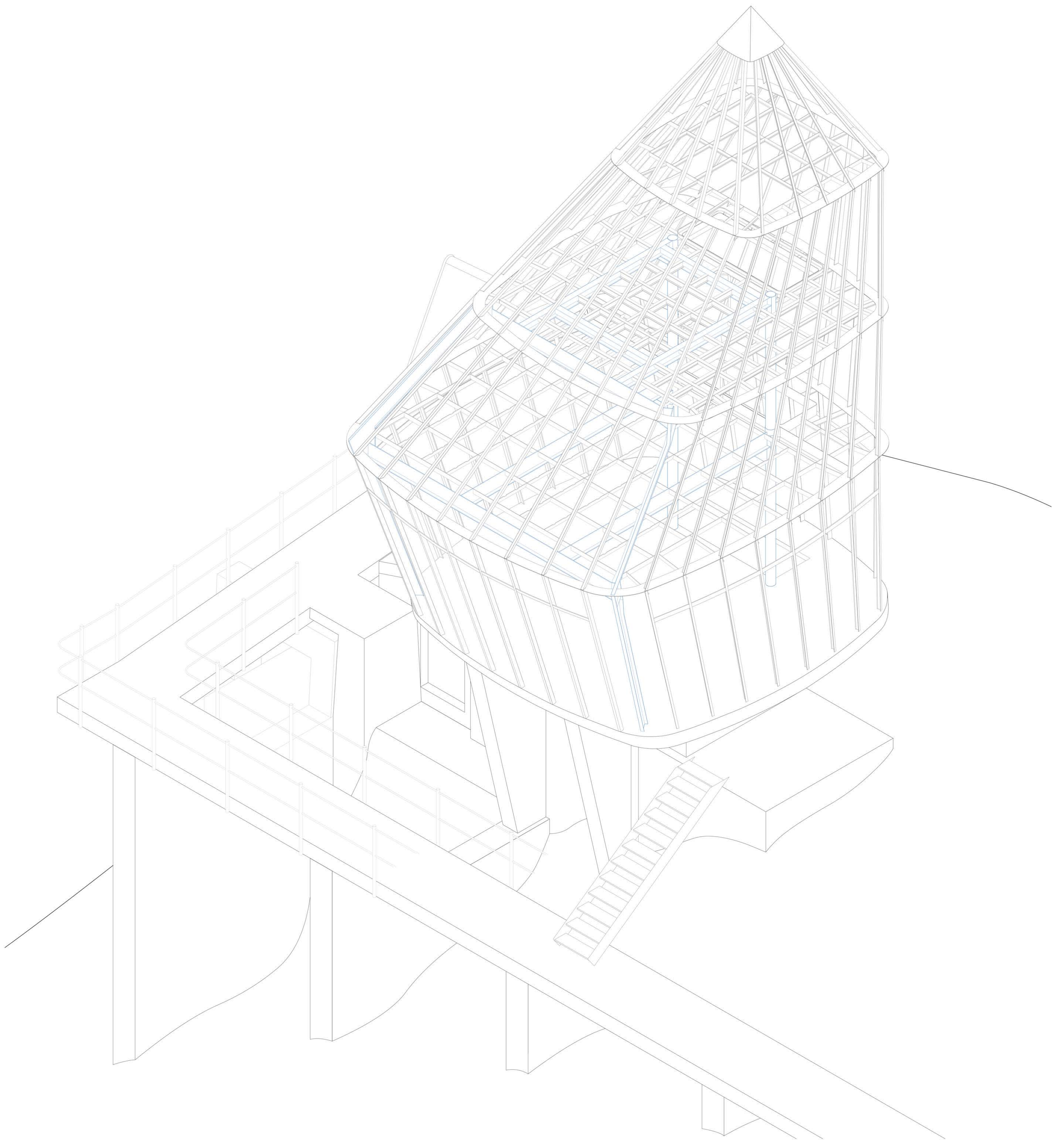
Axonometrie Tragstruktur | 1:20
