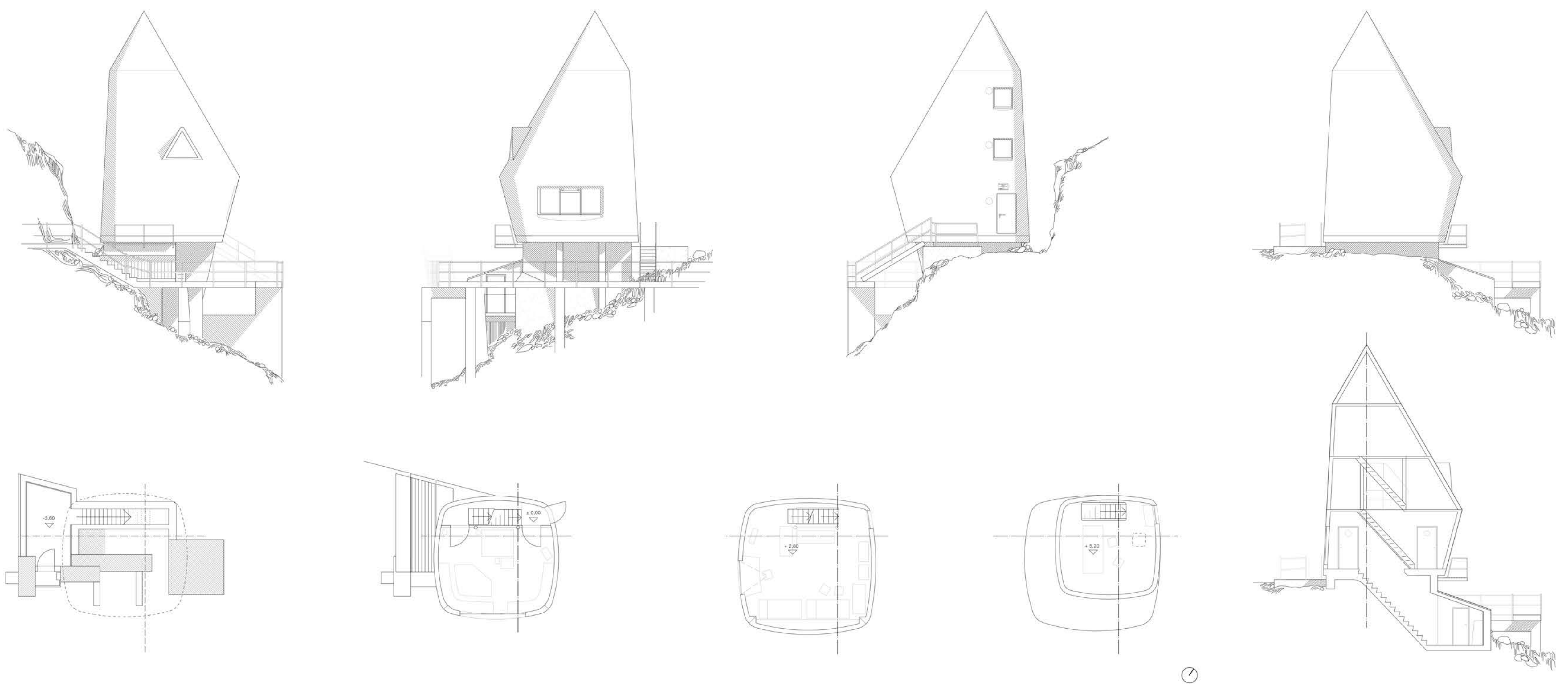
Bestandspläne | 1:100
