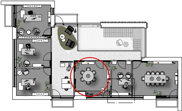
Grundriss OG Übersicht M. 1:300
