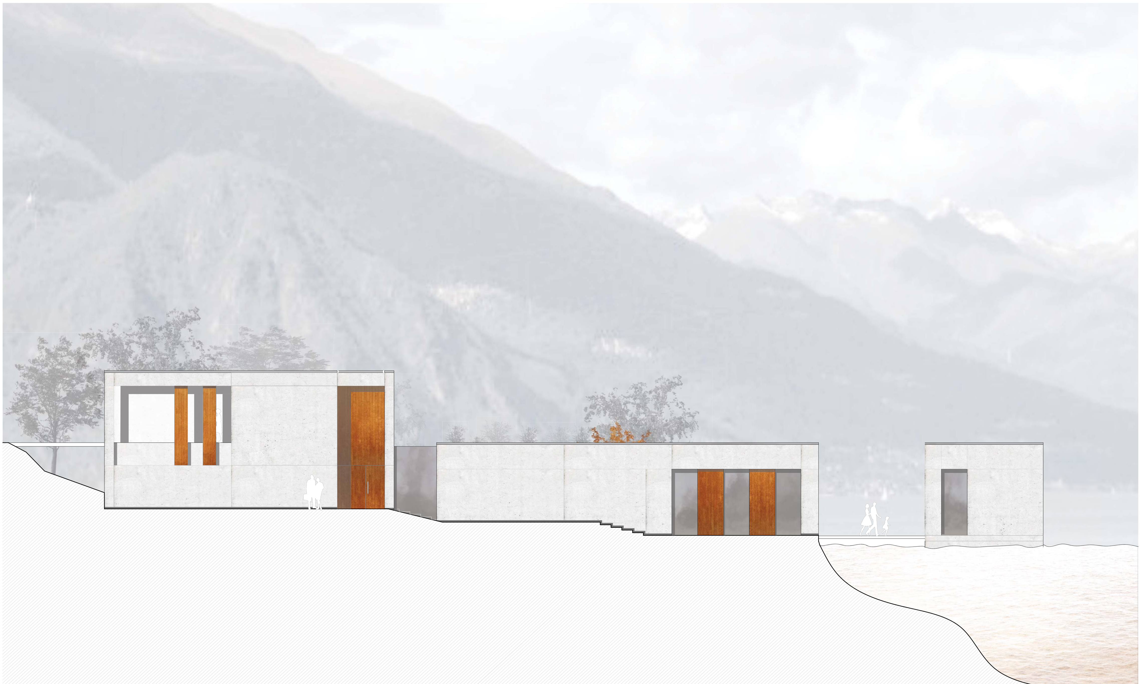
Ansicht Süd | M 1:100
