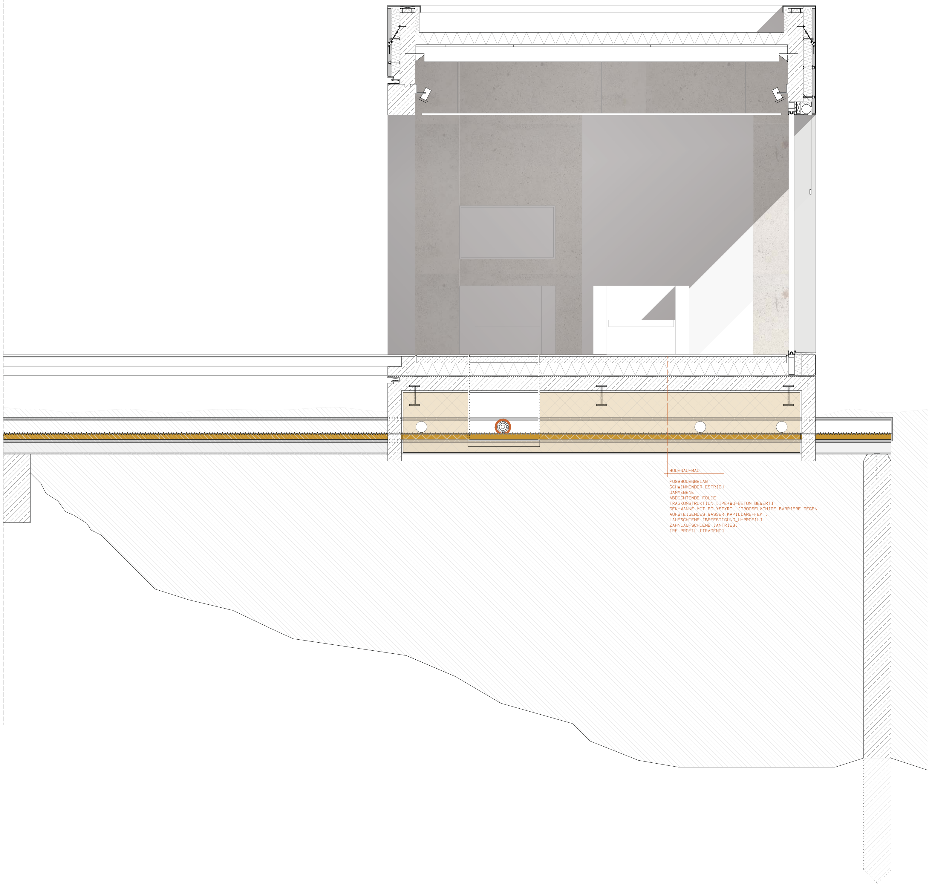
Querschnitt vorderer Gebäudeteil | M 1:33
