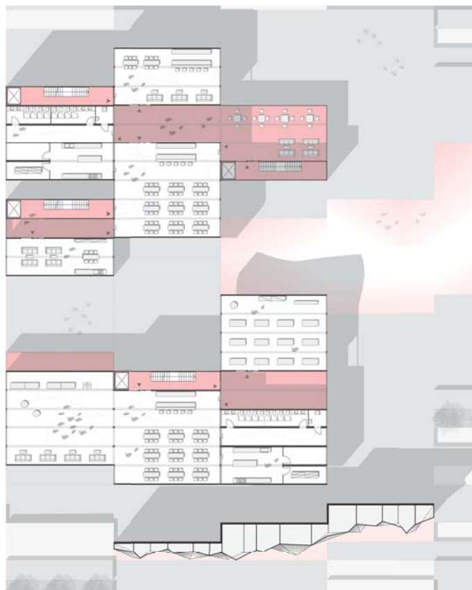
1. OG _ M 1:200
