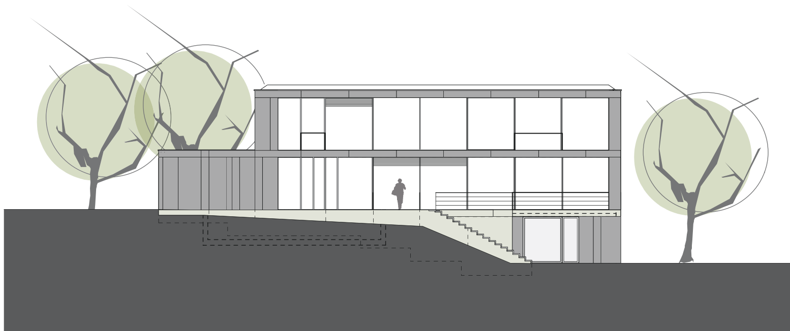
Ansicht Süd
