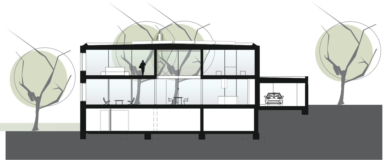
Schnitt AA
