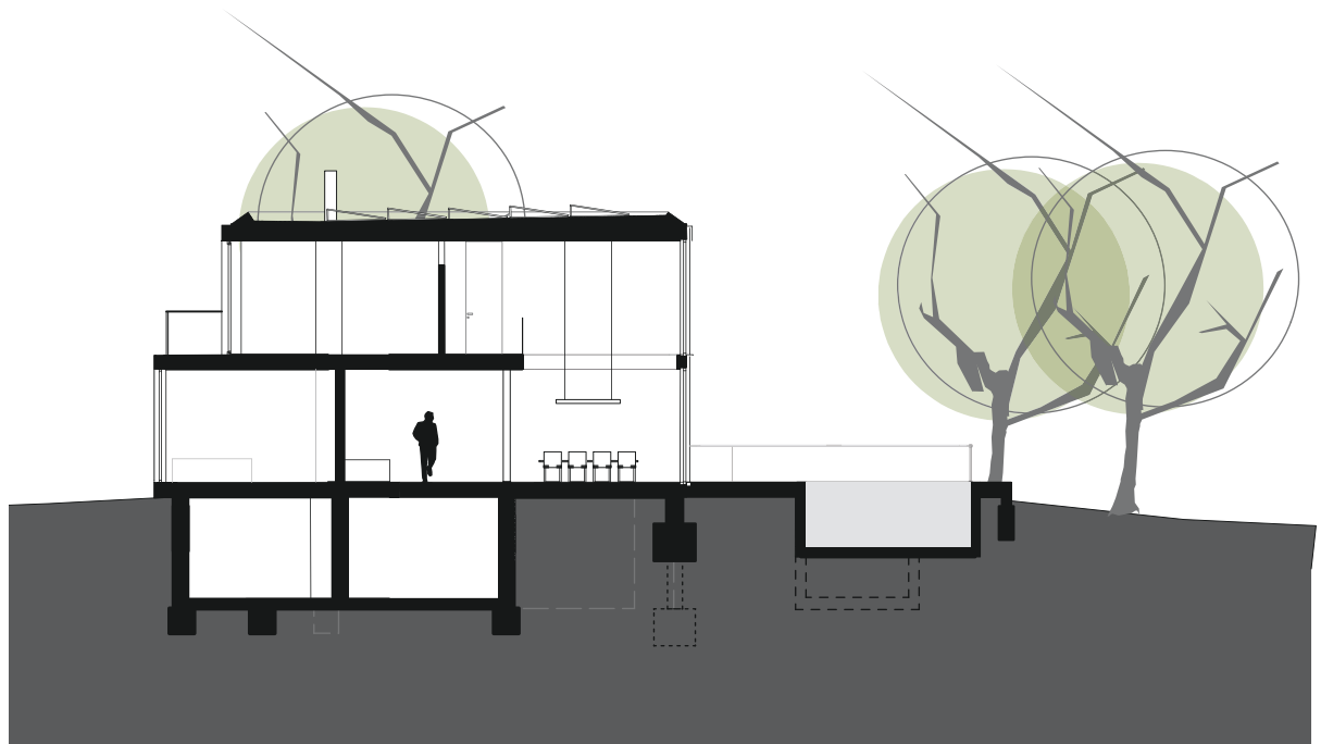
Schnitt BB
