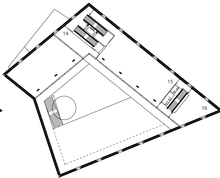
2. Obergeschoss
