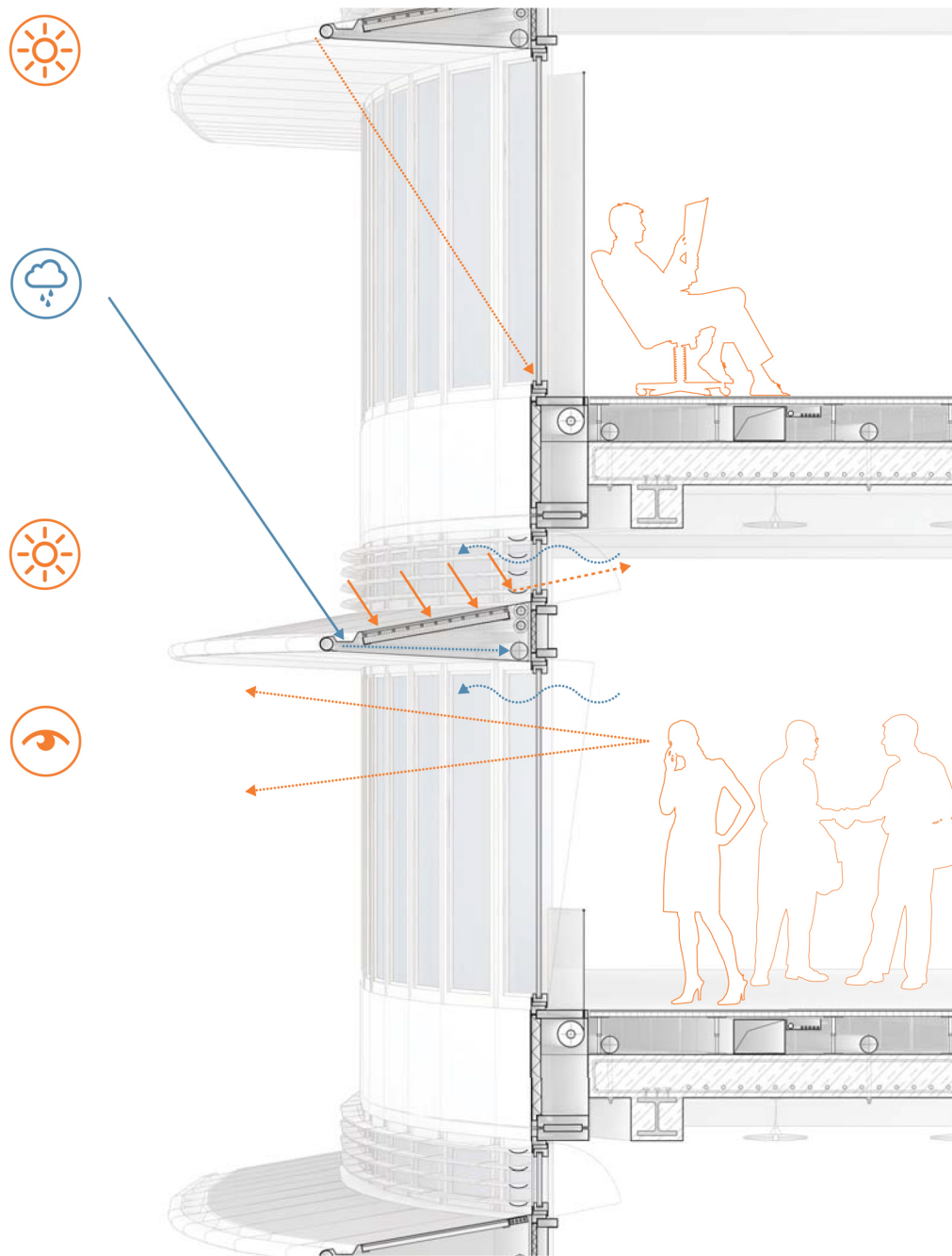
Elementfassade | Schnitt durch Arbeitsbereich
