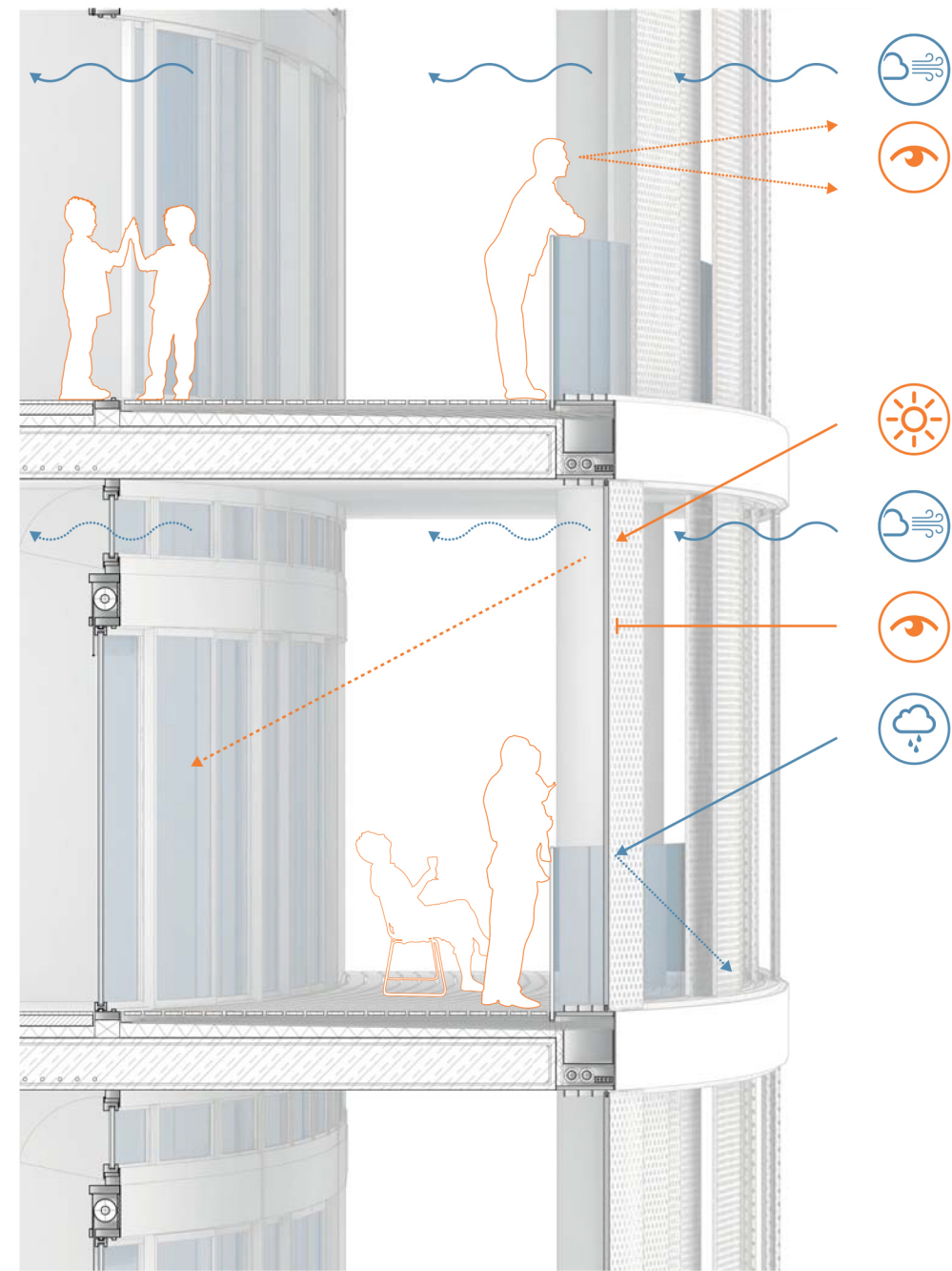
Pfosten-Riegel Fassade | Schnitt durch Wohnbereich
