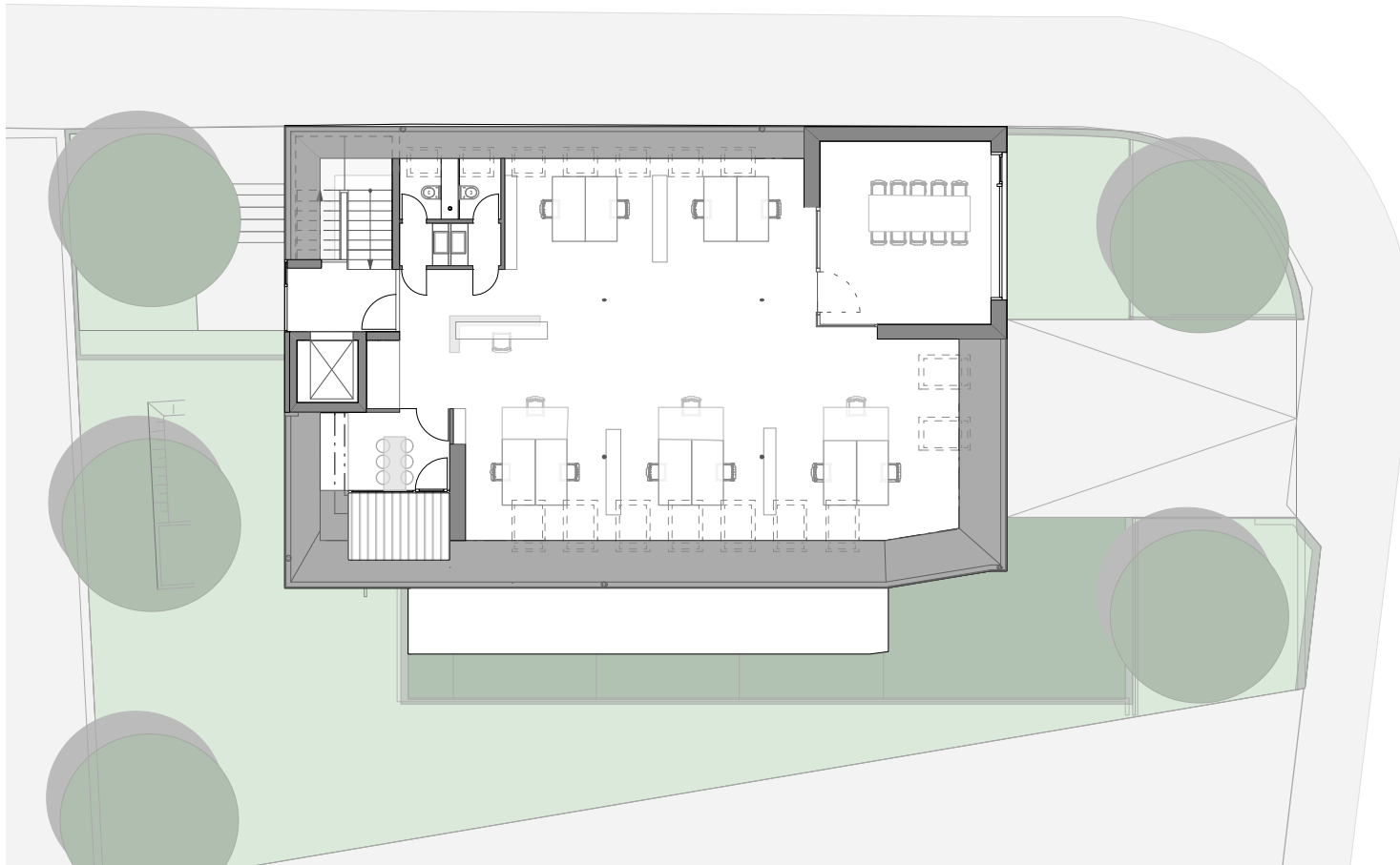
Grundriss DG M 1:200
