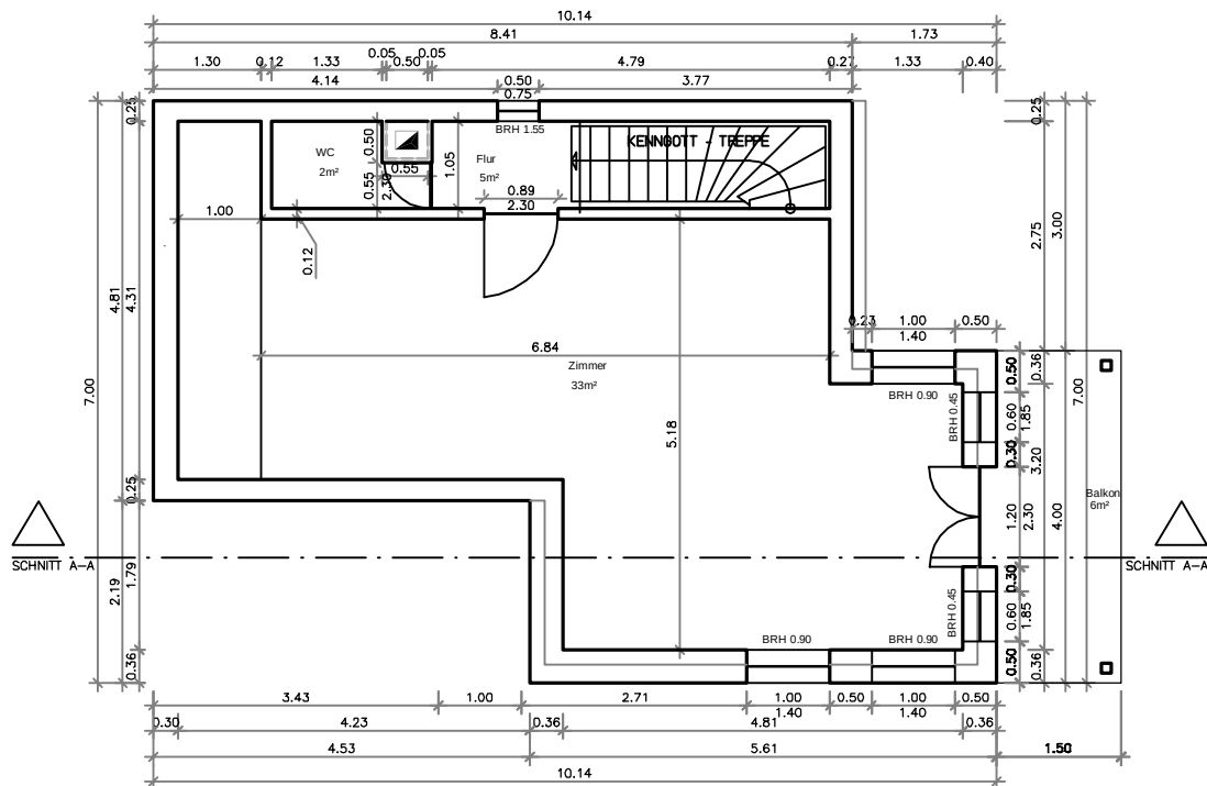
GRUNDRISS DG
