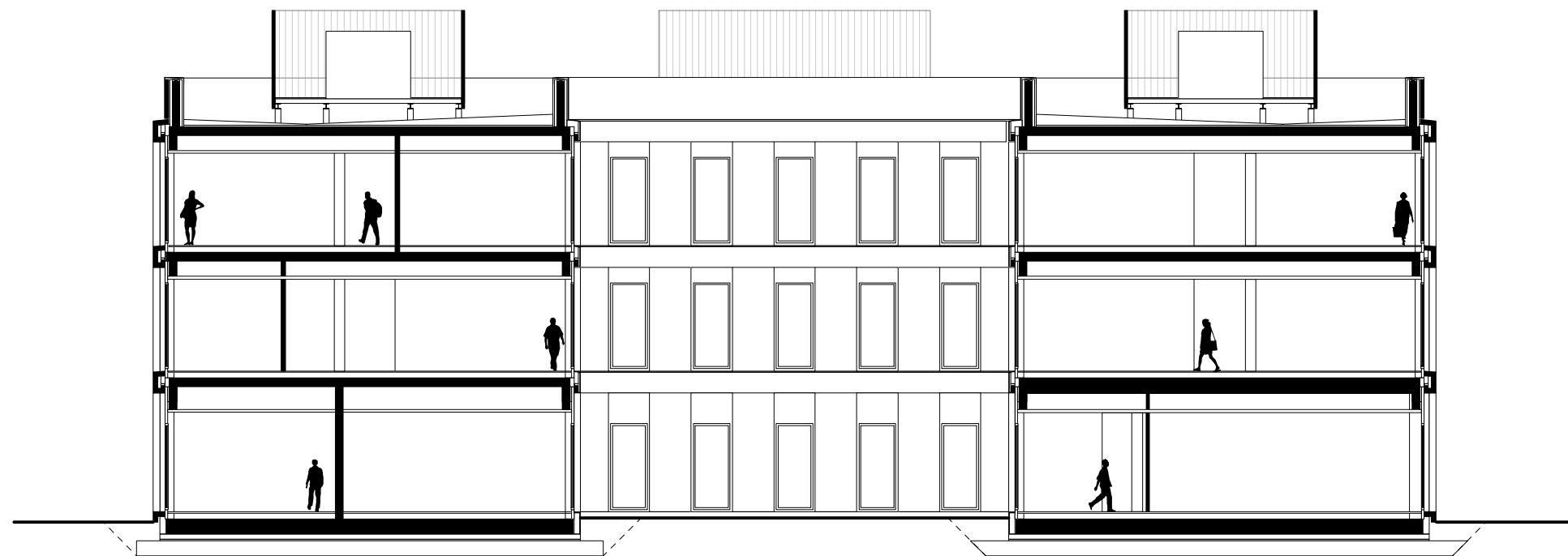
Schnitt C-C / Section C-C
