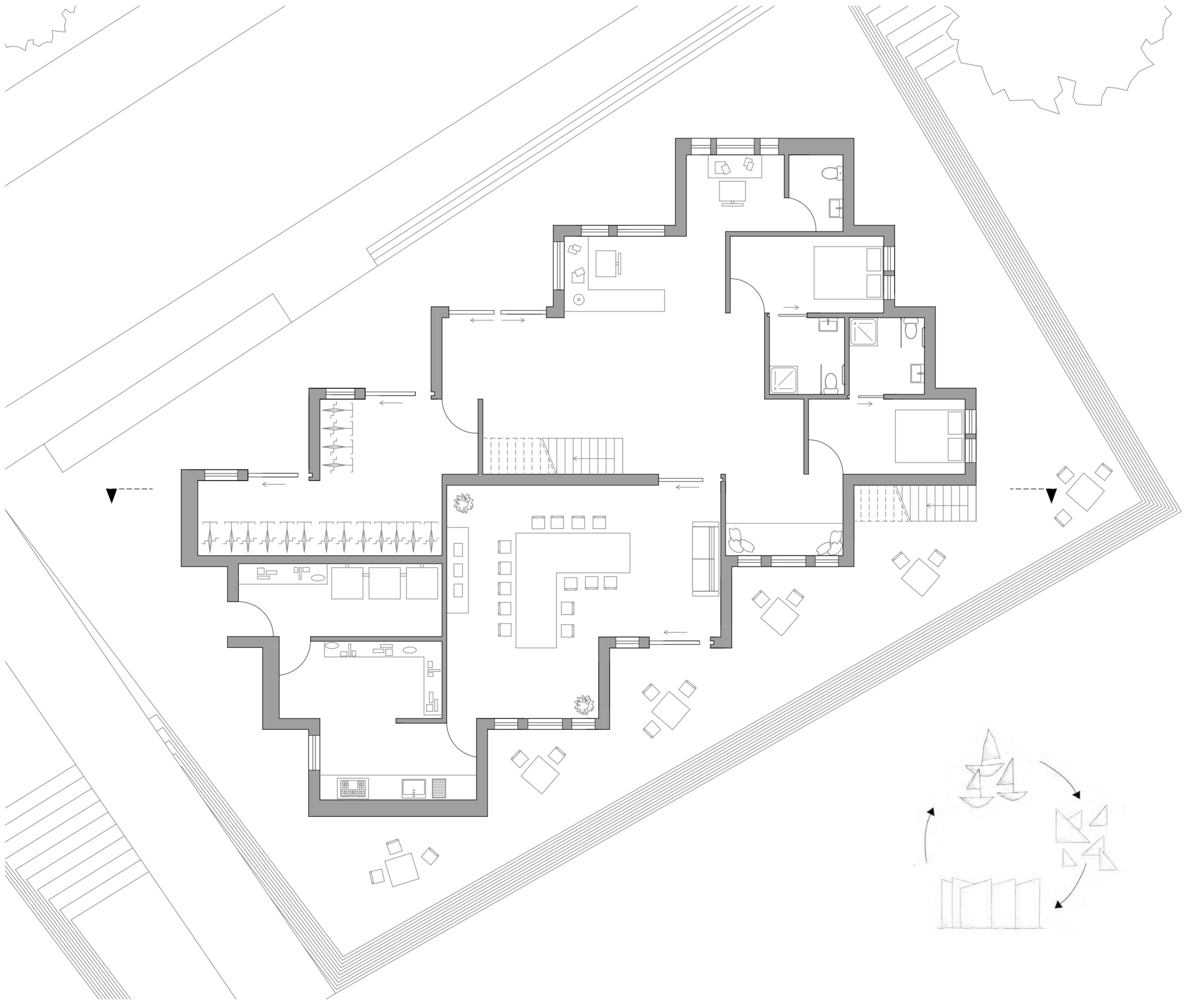
Grundriss EG | 1:100 0 1 2 5
