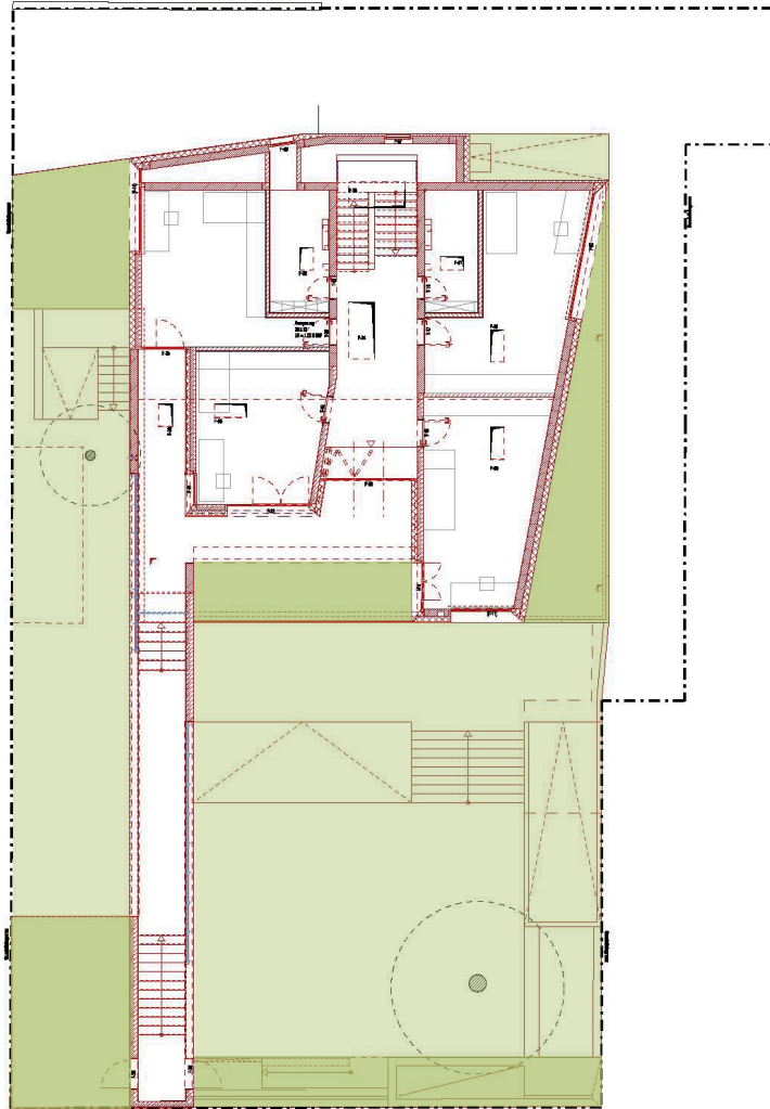
GRUNDRISS OBERGESCHOSS
