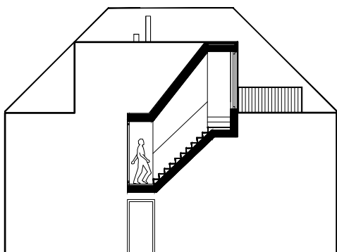
Schnitt CC
