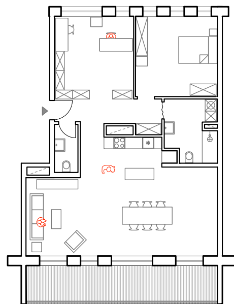
WE 0-03 3-Zi.-Whg. mit großzügigem Wohnbe- reich
