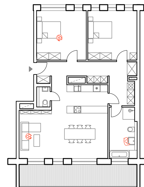
WE 5-03 3 Zi.-Whg. mit Wohnküche und Tageslichtbad
