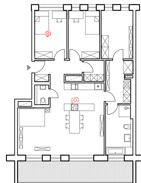
WE 5-02 4.-Zi.-Wg mit großem Hauswirtschaftsbereich
