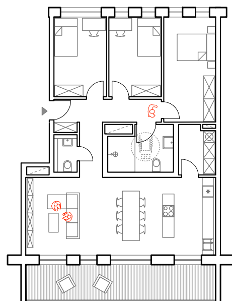
WE 5-01 4-Zi.-Familienwhg. mit Speisekammer
