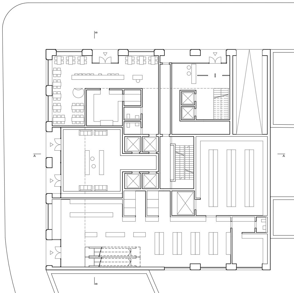
Grundriss Erdgeschoss 1:200
