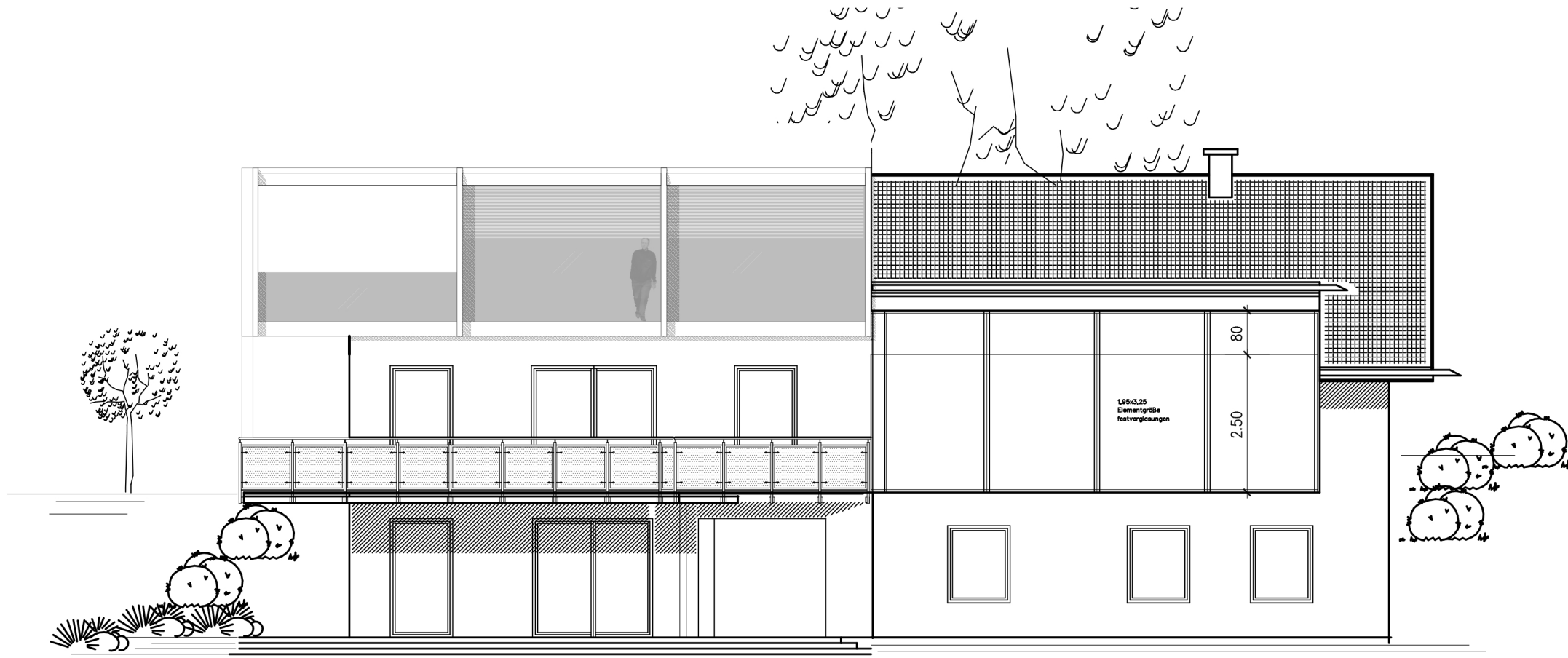
Ansicht Ost
