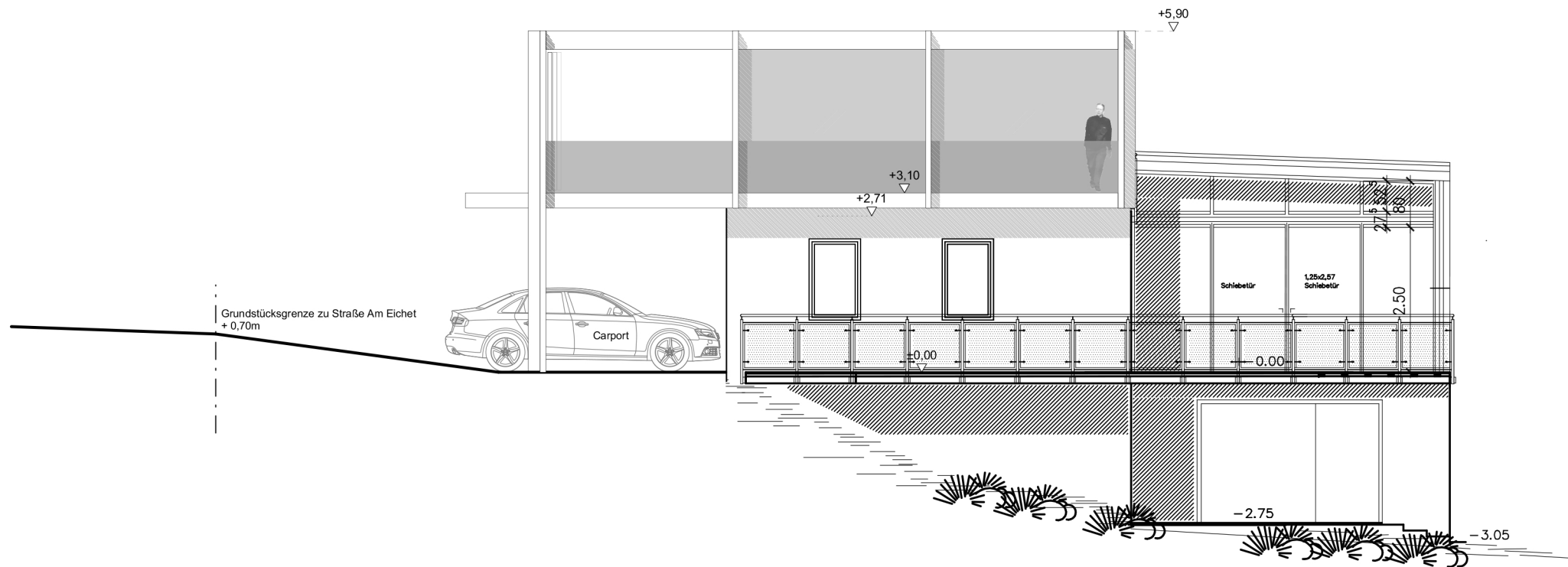
Ansicht Süd
