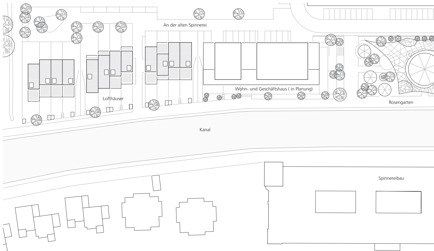
Lofthäuser an der alten Spinnerei Kolbermoor Lageplan
