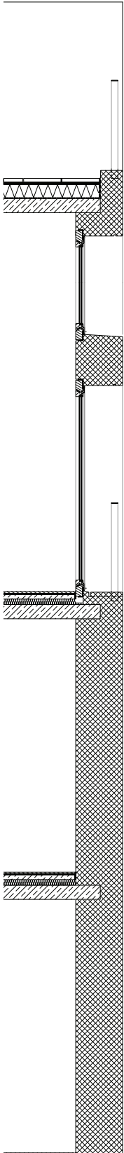
Detailsschnitt M 1:20
