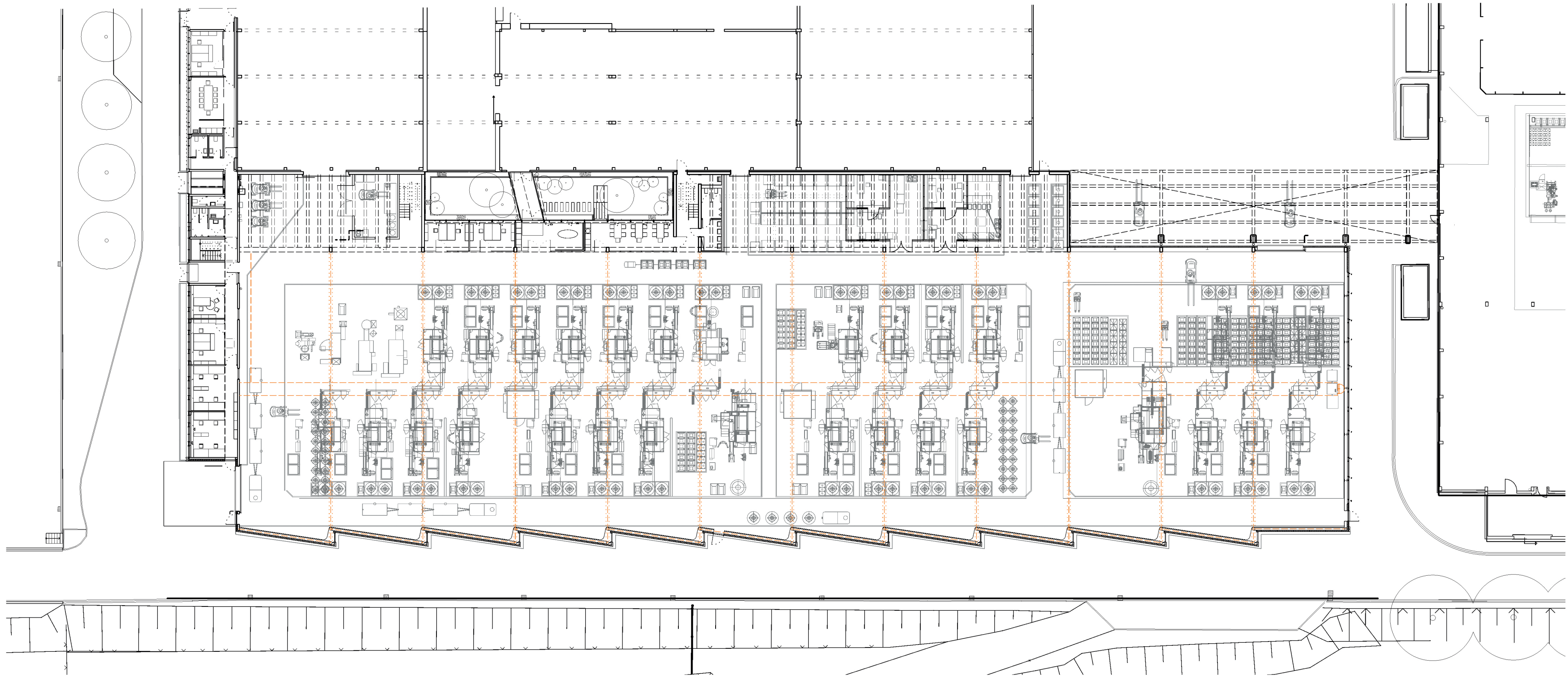
GRUNDRISS, M 1:350
