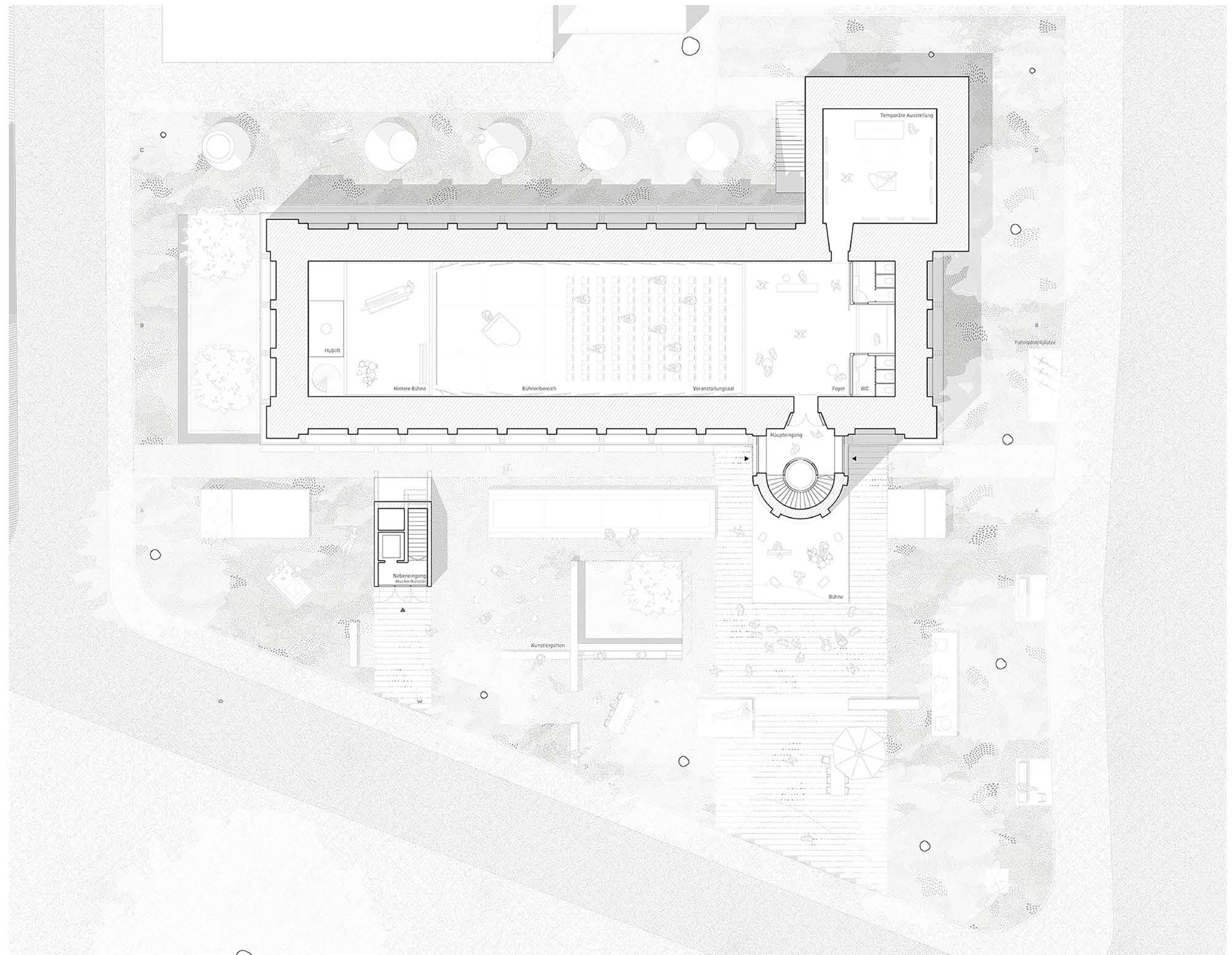
Grundriss Erdgeschoss
