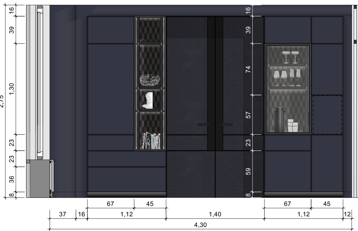
ANSICHT C | M 1:33
