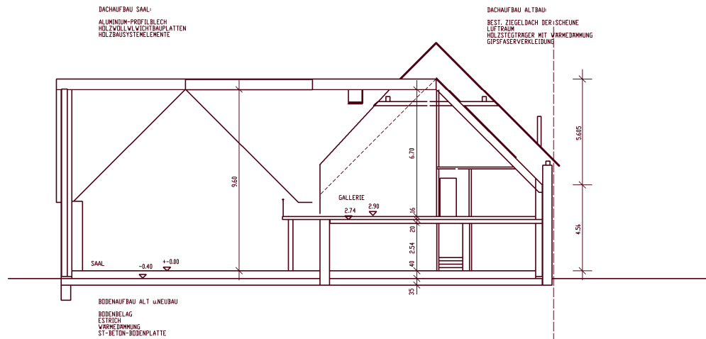
SCHNITT C-C
