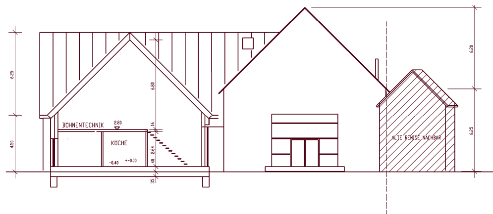
SCHNITT A-A
