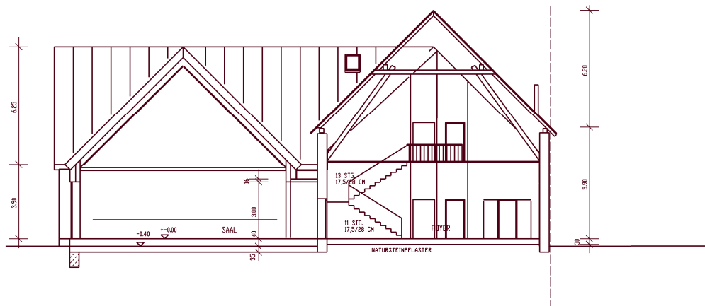
SCHNITT B-B
