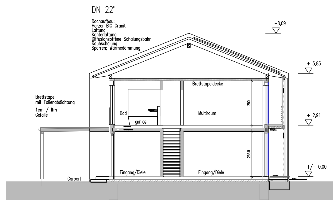
Quer-Schnitt
