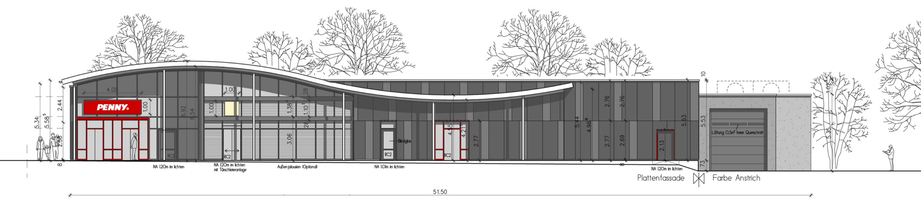
ANSICHT VON DER STRASSE AM ALTEN FÄHRHAUS
