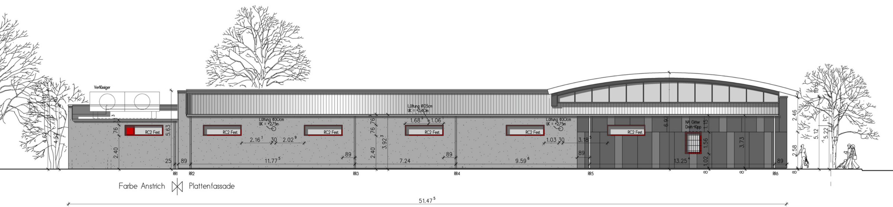
ANSICHT VON NORD—WEST
