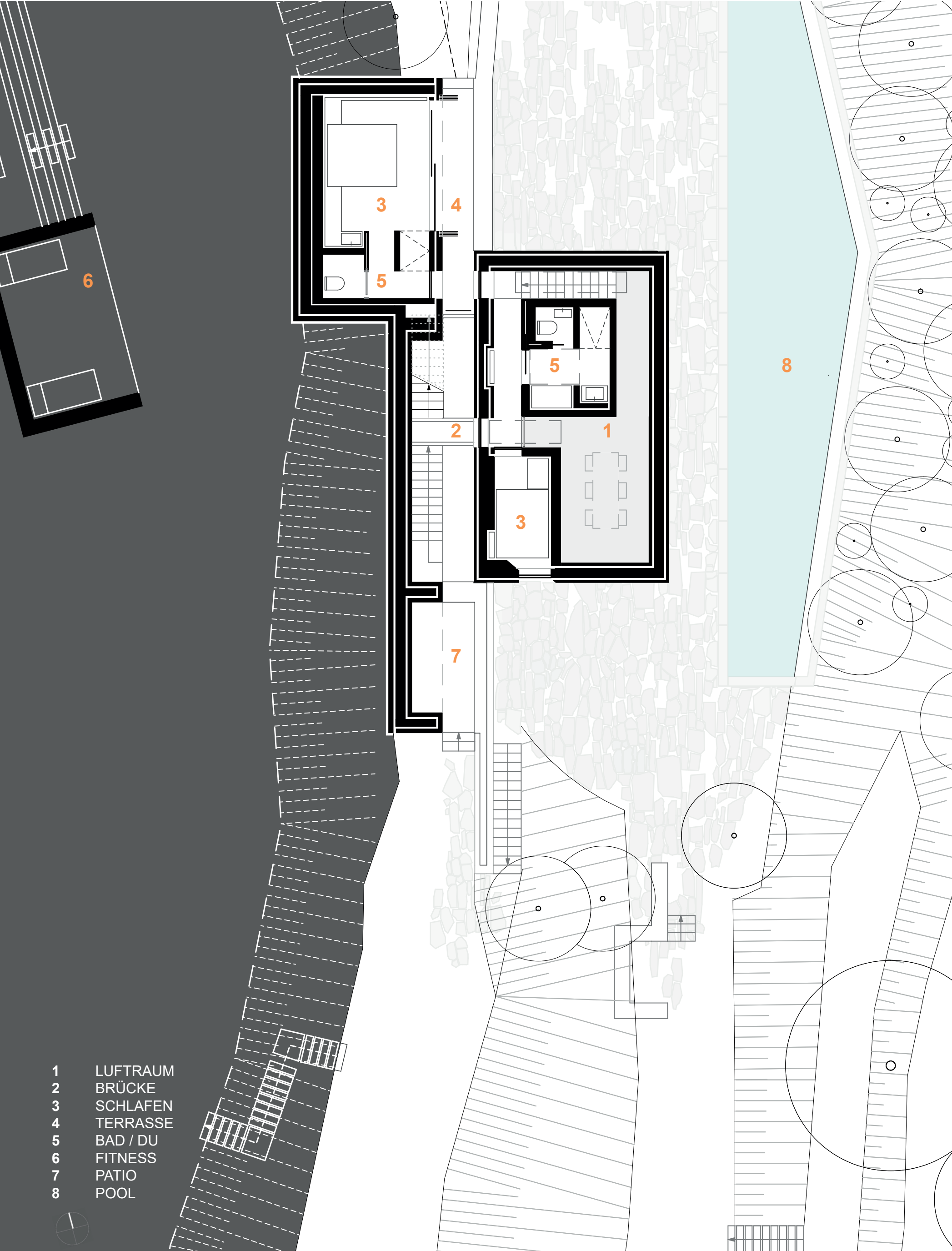
RUSTICO GARGNANO GARDASEE GRUNDRISS OG M 1:100
