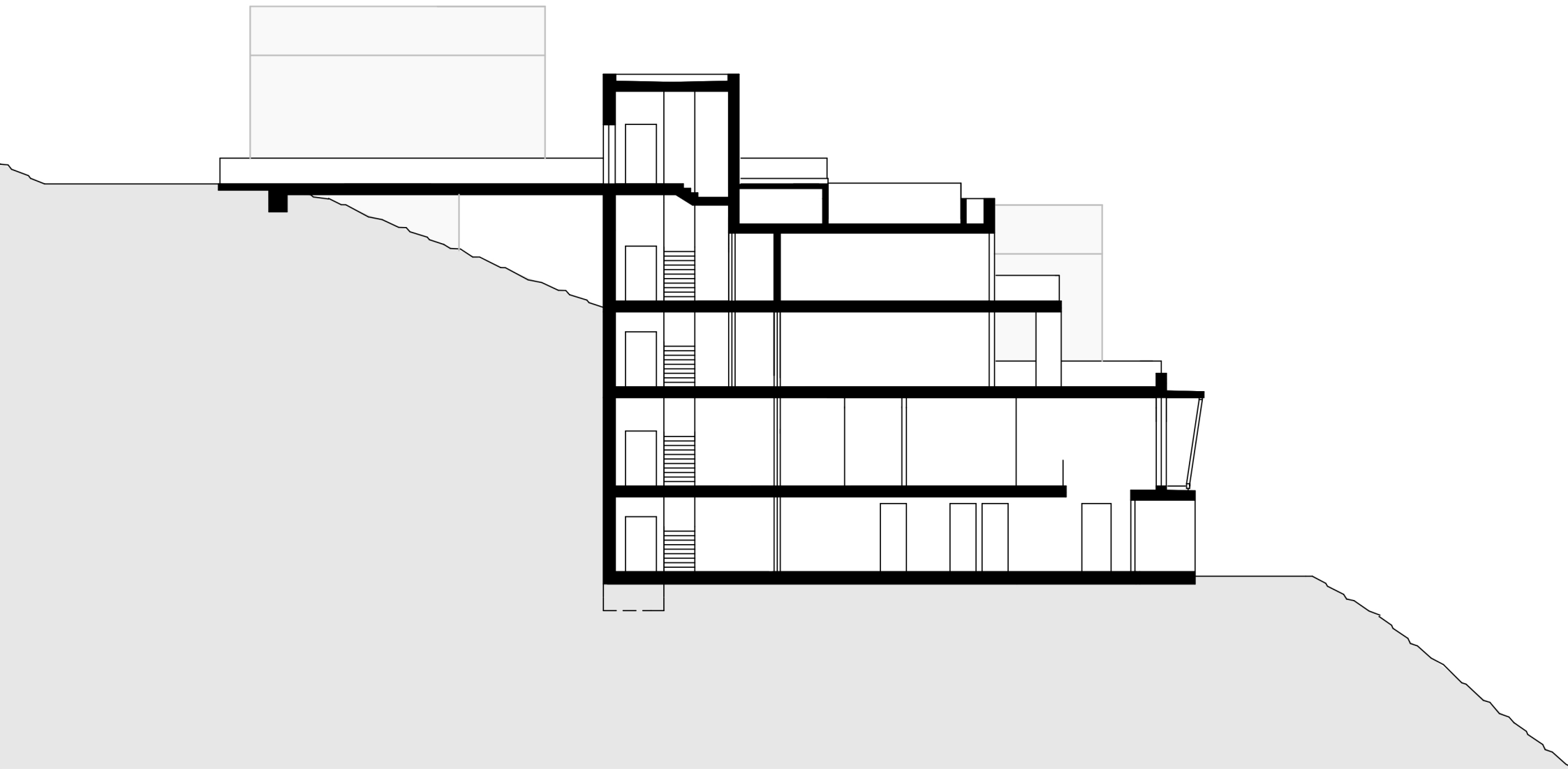
Schnitt Zentralgebäude
