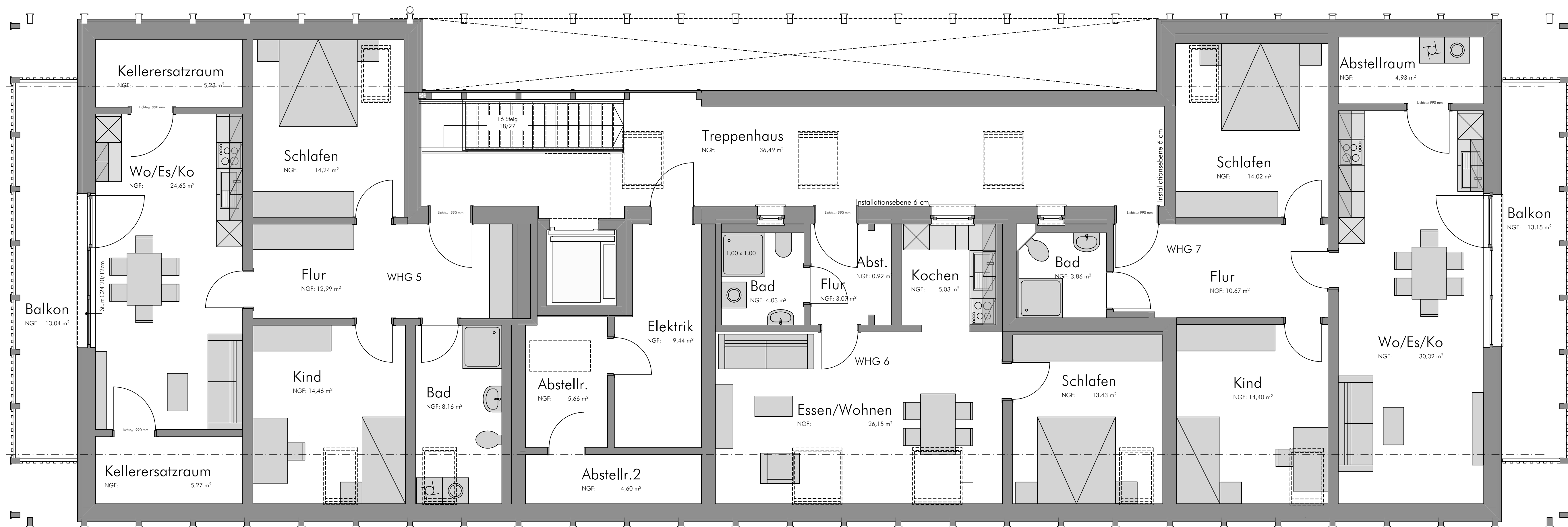
Grundriss Dachgeschoss
