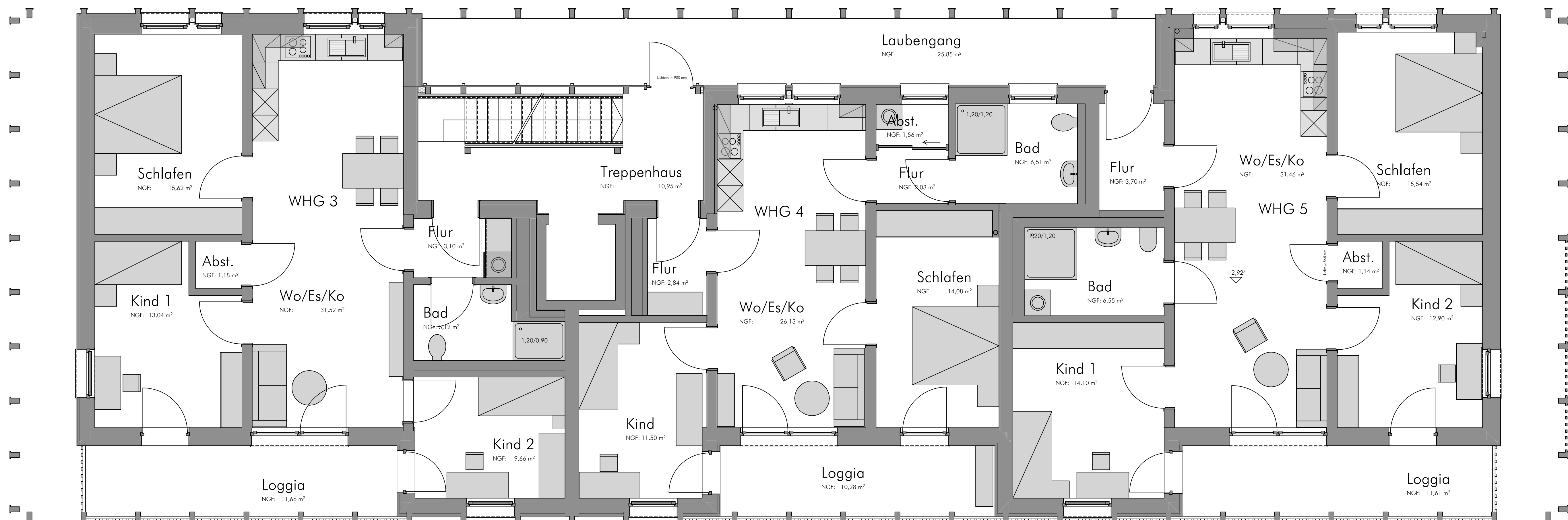
Grundriss Obergeschoss
