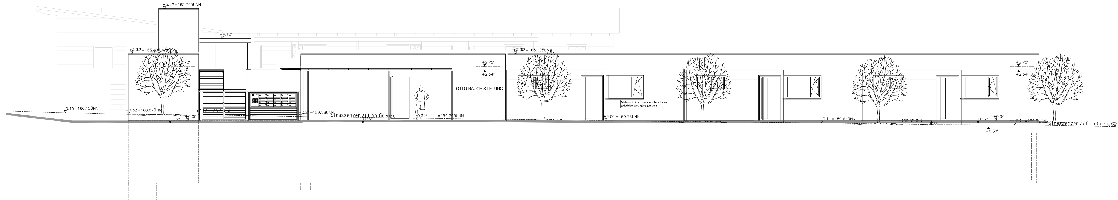
Nordostansicht M 1:100
