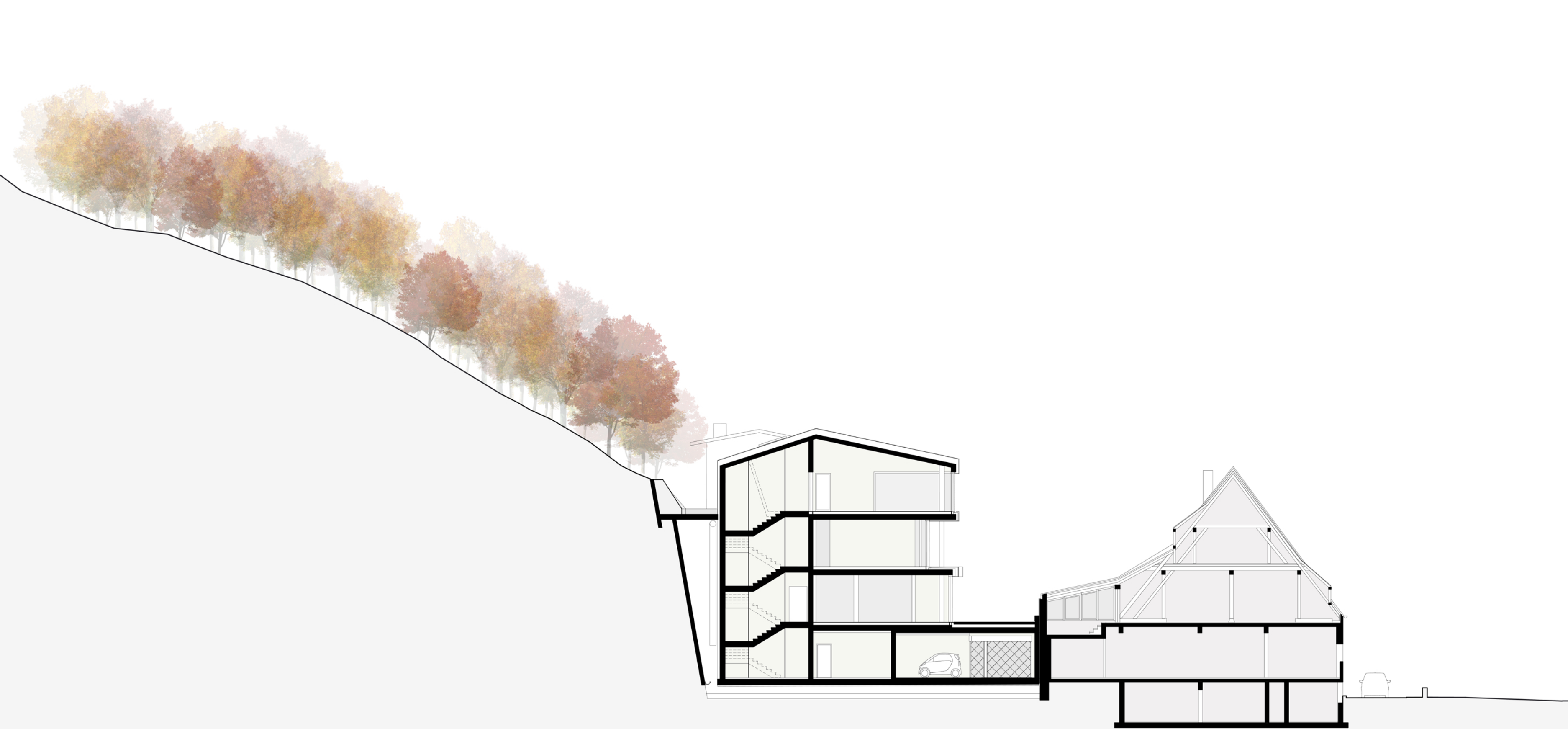
Schnitt A-A M 1:200
